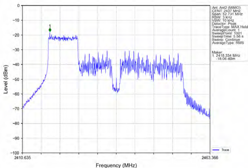
802.11ax(HE40) MCH 2437MHz RU106 Left MIMO NTN
