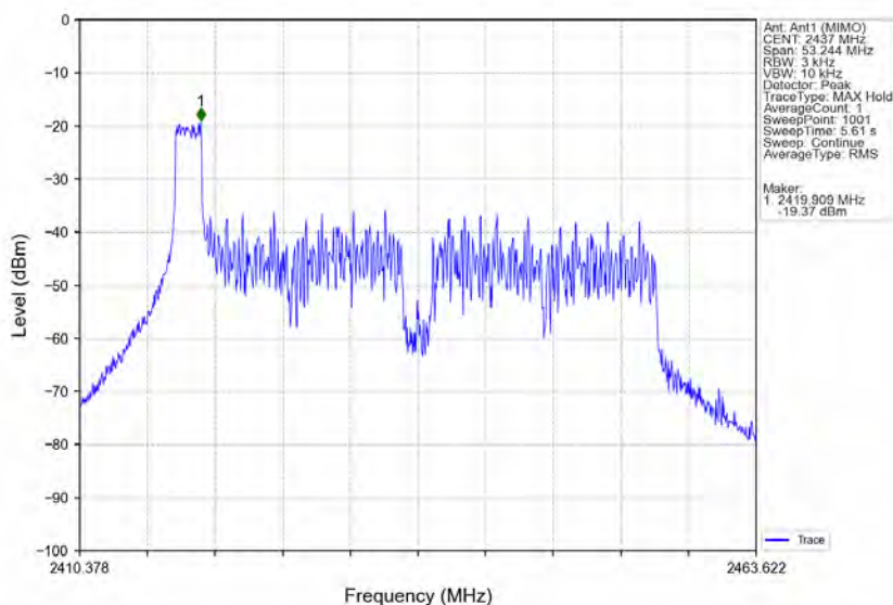
802.11ax(HE40) MCH 2437MHz RU26 Left Ant1 (MIMO) NTVN
