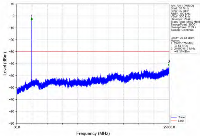
802.11ax(HE20) HCH 2462MHz RU242 Left Ant1 (MIMO) NTNV
