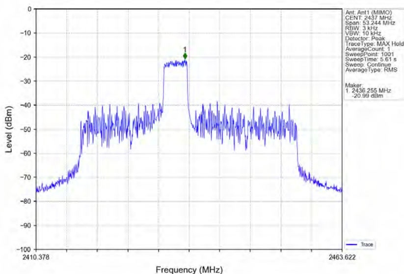
802.11ax(HE40) MCH 2437MHz RU52 Mid Ant1 (MIMO) NTN
