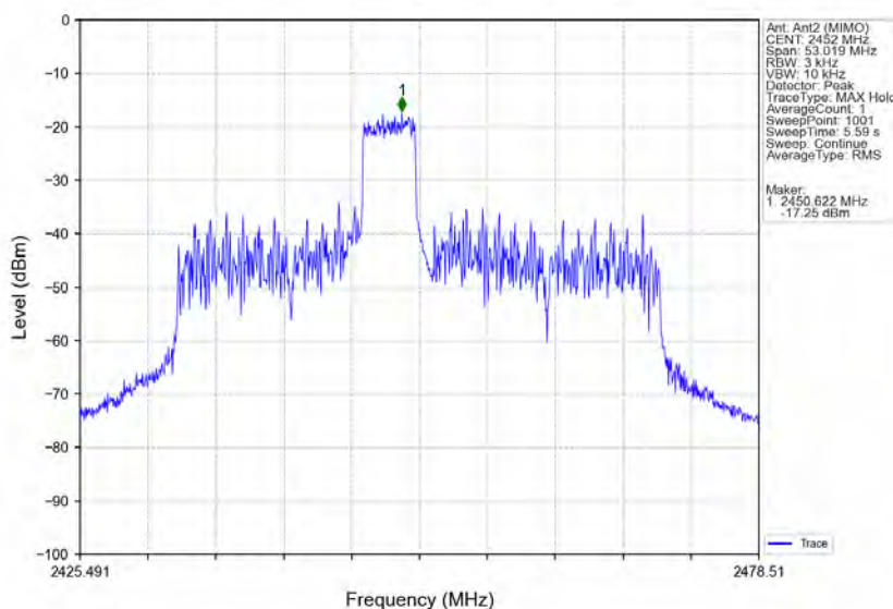
802.11ax(HE40) HCH 2452MHz RU52 Mid MIMO NTNV
