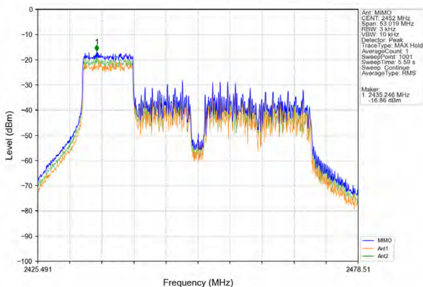
802.11ax(HE40) HCH 2452MHz RU106 Left MIMO NTN
