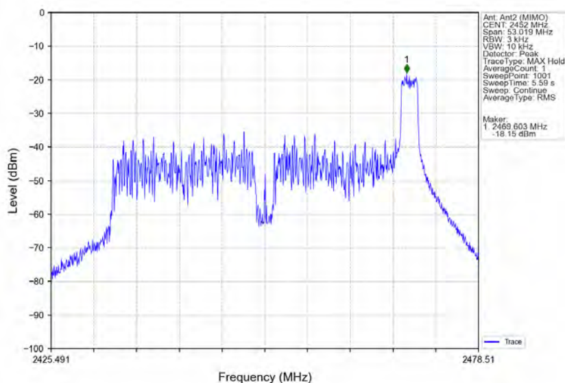
802.11ax(HE40) HCH 2452MHz RU26 Right MIMO NTN
