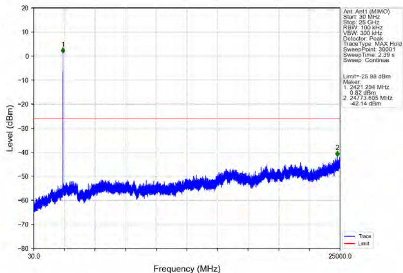
802.11ax(HE20) LCH 2412MHz RU242 Left Ant1 (MIMO) NTVN
