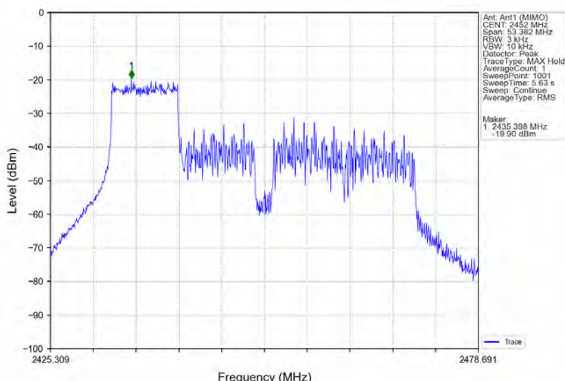
802.11ax(HE40) HCH 2452MHz RU106 Left Ant1 (MIMO) NTNV
