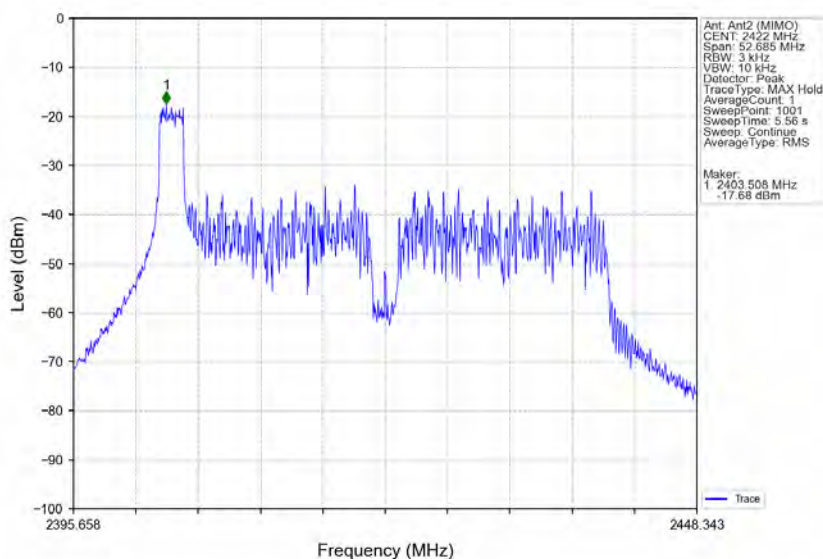
802.11ax(HE40) LCH 2422MHz RU26 Left MIMO NTNV
