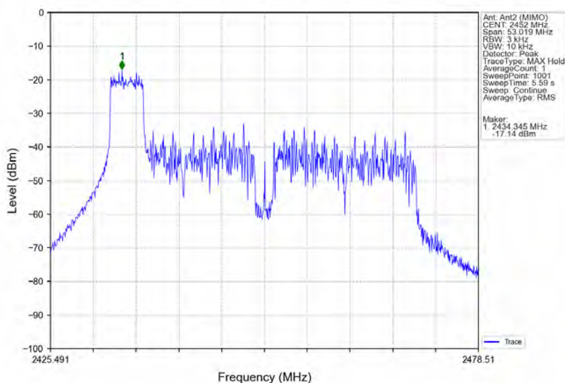
802.11ax(HE40) HCH 2452MHz RU52 Left Ant2 (MIMO) NTVN
