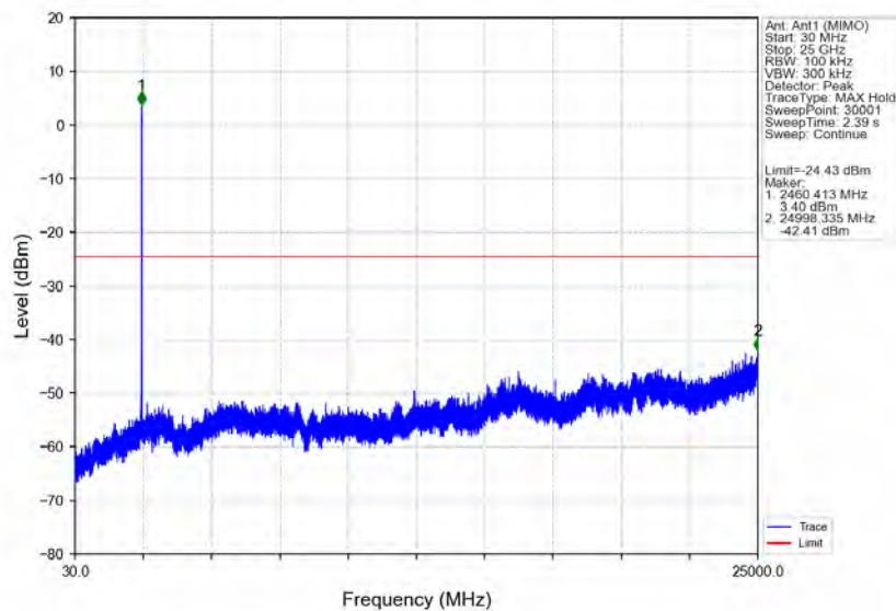
802.11b HCH 2462MHz Ant1 (MIMO) NTN
