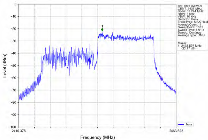
802.11ax(HE40) MCH 2437MHz RU242 Right Ant1 (MIMO) NTN
