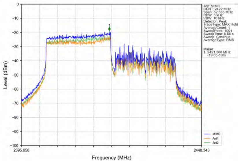
802.11ax(HE40) LCH 2422MHz RU242 Right Ant1 (MIMO) NTN
