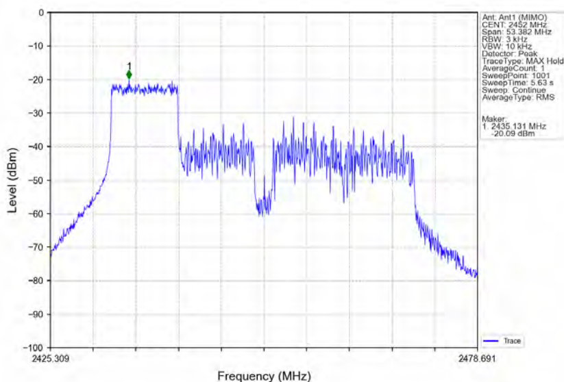
802.11ax(HE40) HCH 2452MHz RU106 Right Ant1 (MIMO) NTN
