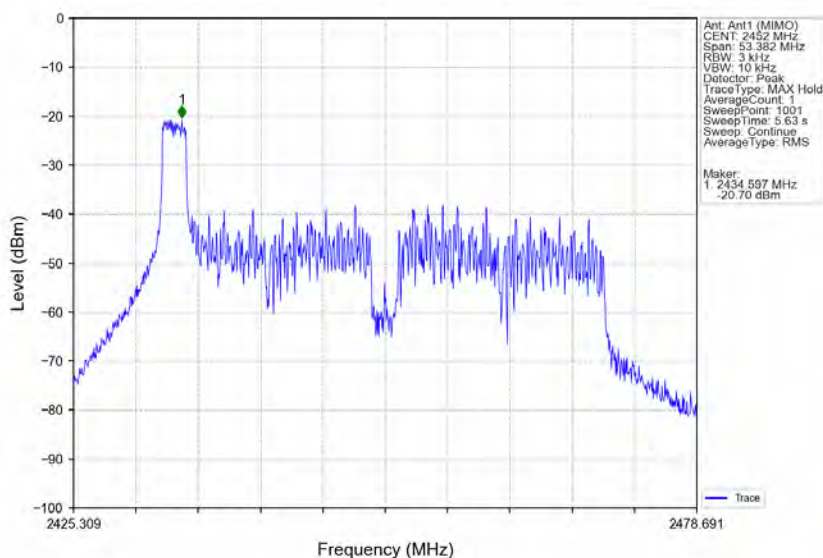
802.11ax(HE40) HCH 2452MHz RU26 Left Ant1 (MIMO) NTV
