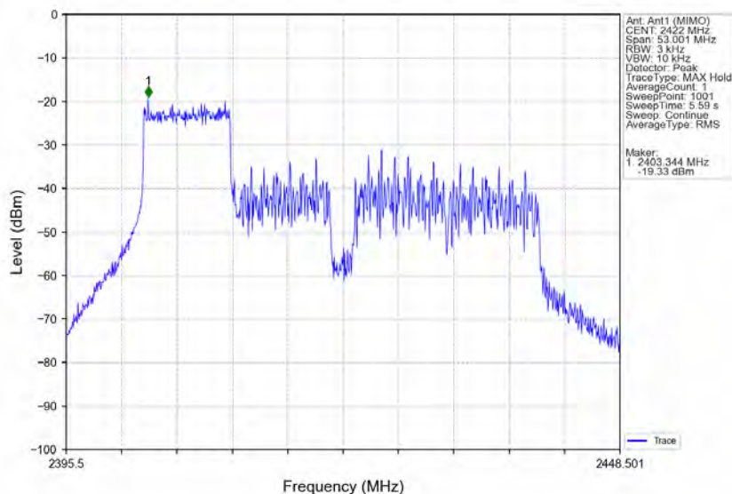
802.11ax(HE40) LCH 2422MHz RU106 Left Ant1 (MIMO) NTVN
