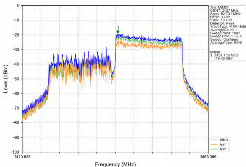
802.11ax(HE40) MCH 2437MHz RU242 Right MIMO NTN
