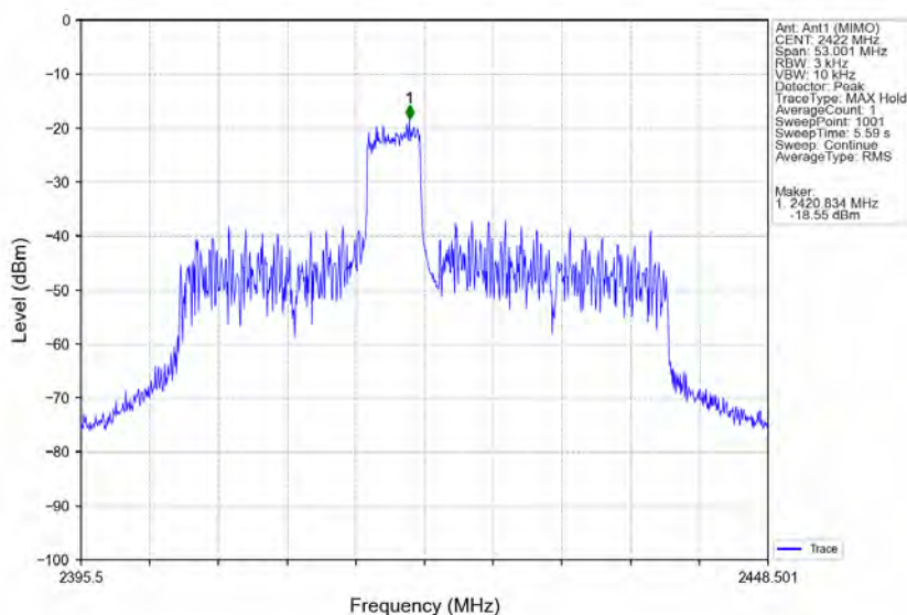
802.11ax(HE40) LCH 2422MHz RU52 Mid Ant1 (MIMO) NTN
