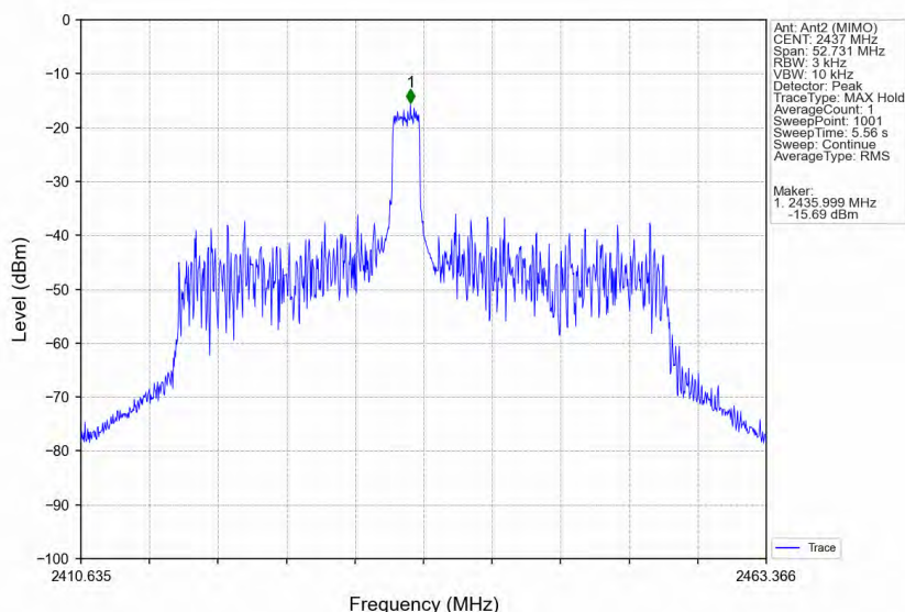
802.11ax(HE40) MCH 2437MHz RU26 Right MIMO NTN
