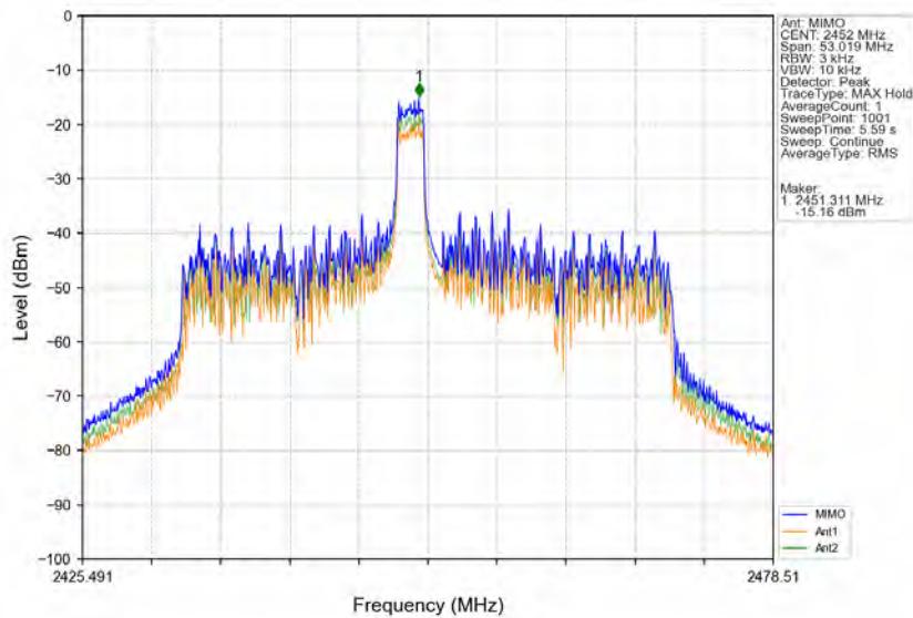
802.11ax(HE40) HCH 2452MHz RU26 Right Ant1 (MIMO) NTNv
