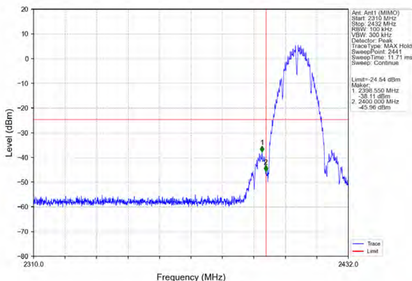
802.11b_LCH_2412MHz_Ant1 (MIMO)_NTNV
