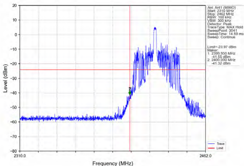
802.11ax(HE40) LCH 2422MHz RU484 Left Ant1 (MIMO) NTNV
