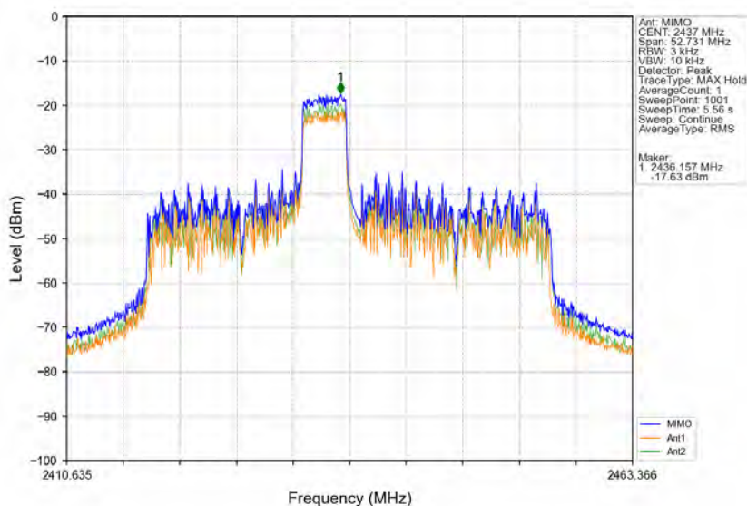
802.11ax(HE40) MCH 2437MHz RU52 Mid MIMO NTNV
