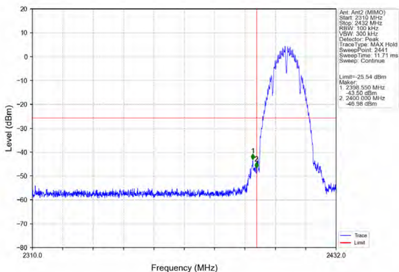
802.11b LCH 2412MHz Ant2 (MIMO) NTN
