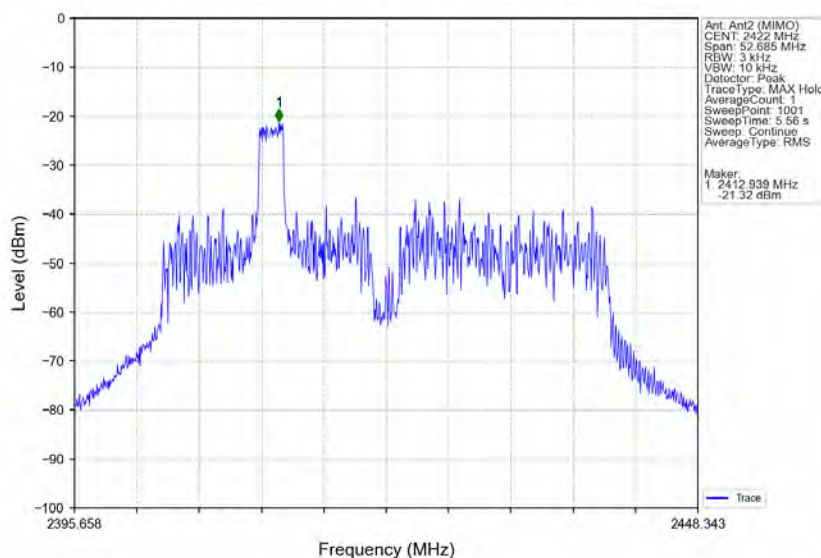
802.11ax(HE40) LCH 2422MHz RU26_Mid Ant2 (MIMO) NTN
