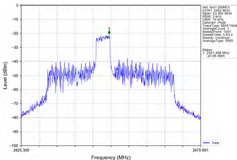
802.11ax(HE40) HCH 2452MHz RU52 Mid Ant1 (MIMO) NTVN
