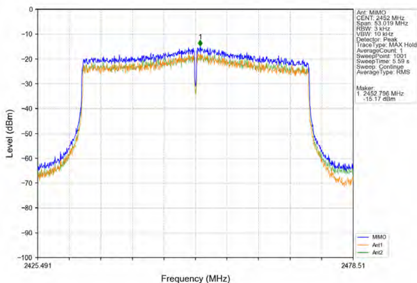
802.11ax(HE40) HCH 2452MHz RU484 Left MIMO NTVN
