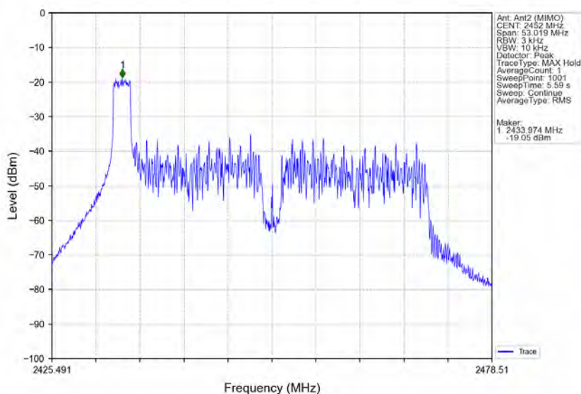
802.11ax(HE40) HCH 2452MHz RU26 Left MIMO NTNV
