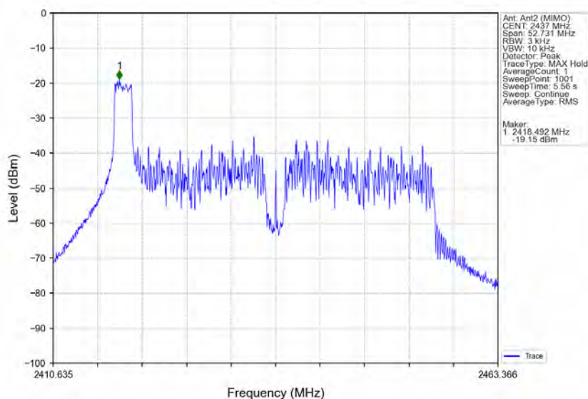
802.11ax(HE40) MCH 2437MHz RU26 Left MIMO NTNV
