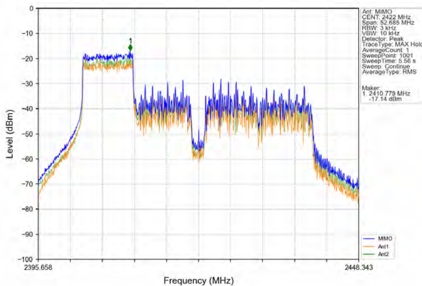
802.11ax(HE40) LCH 2422MHz RU106 Left MIMO NTN
