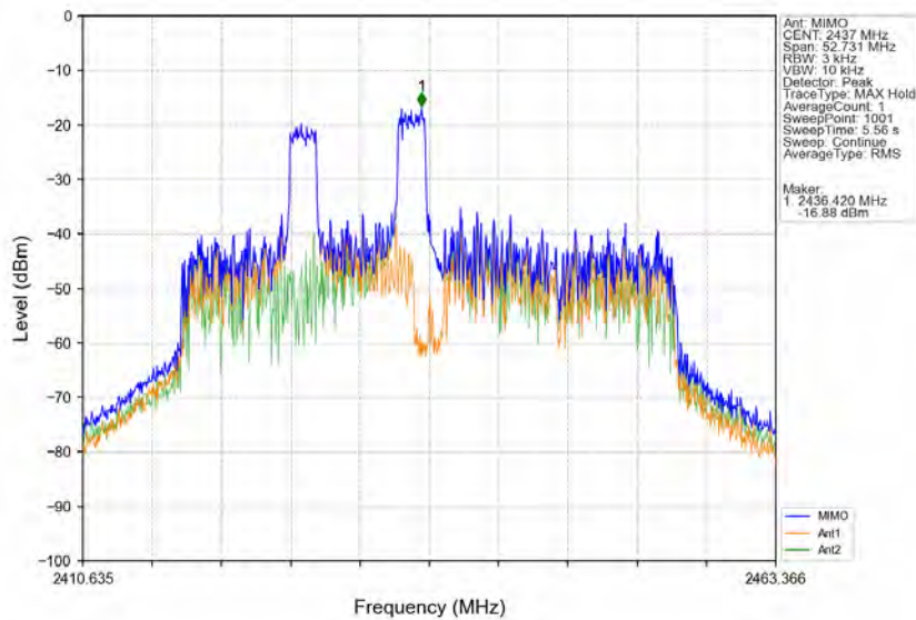
802.11ax(HE40) MCH 2437MHz RU26 Right Ant1 (MIMO) NTN
