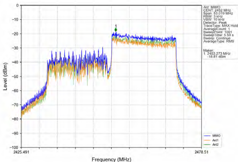
802.11ax(HE40) HCH 2452MHz RU242 Right MIMO NTNv
