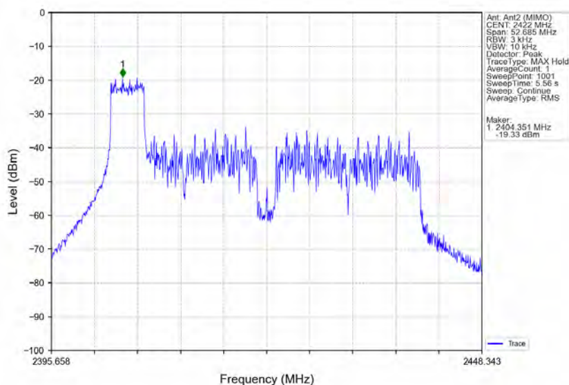
802.11ax(HE40) LCH 2422MHz RU52 Left Ant2 (MIMO) NTV
