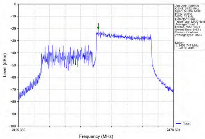
802.11ax(HE40) HCH 2452MHz RU242 Right Ant1 (MIMO) NTN
