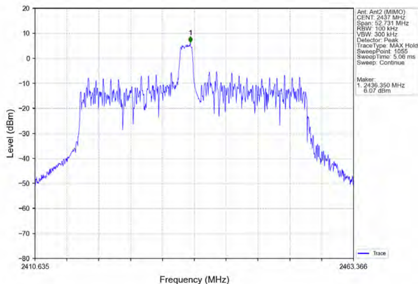
802.11ax(HE40) MCH 2437MHz RU484 Left Ant2 (MIMO) NTNv
