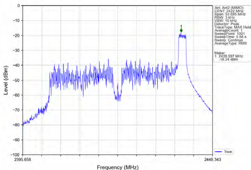
802.11ax(HE40) LCH 2422MHz RU26 Right MIMO NTN
