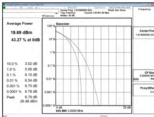
PTAR B25 3M CH26675 64QAM
