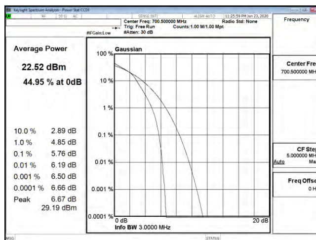
PTAR B12 3M CH23025 16QAM
