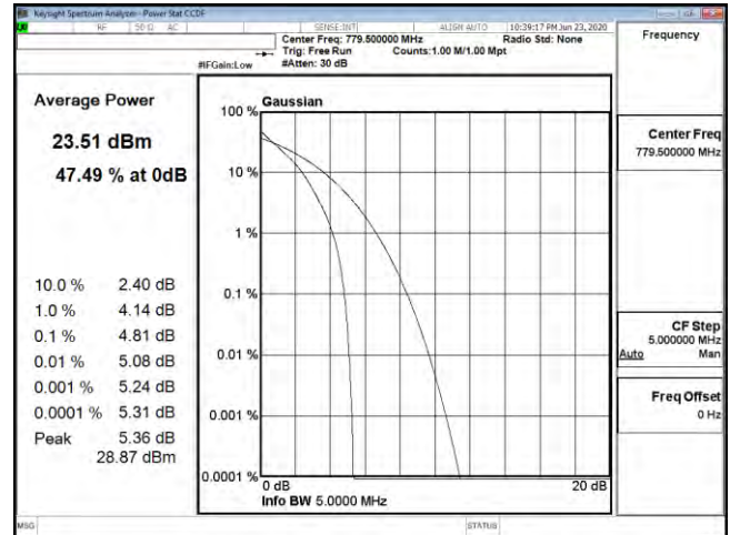
PTAR B13 5M CH23205 QPSK
