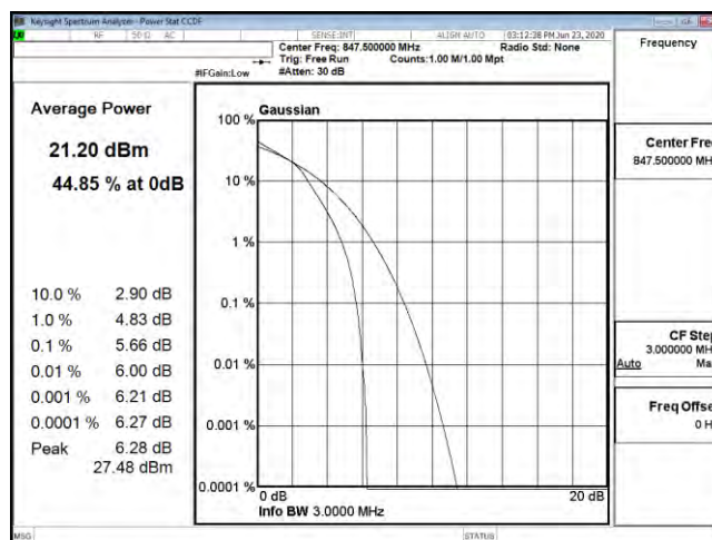
PTAR B26 3M CH27025 16QAM
