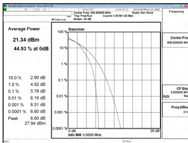
PTAR B26 3M CH26915 16QAM
