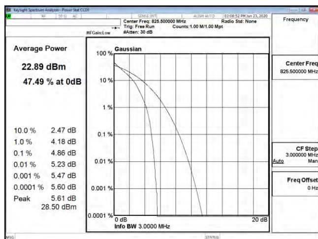
PTAR B26 3M CH26805 QPSK
