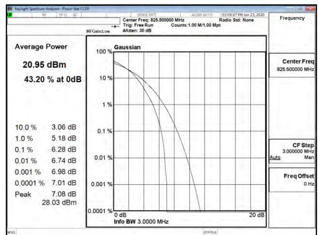
PTAR B26 3M CH26805 64QAM
