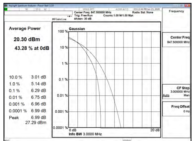
PTAR B26 3M CH27025 64QAM
