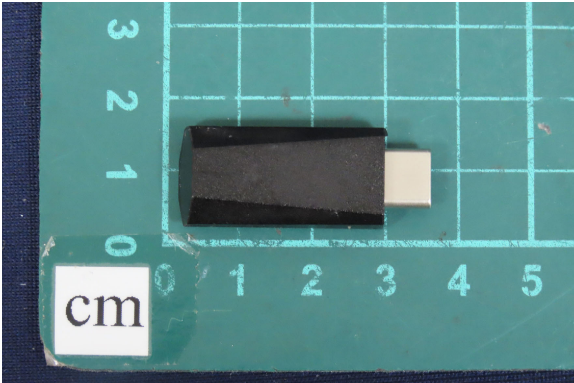
(2) EUT Photo
