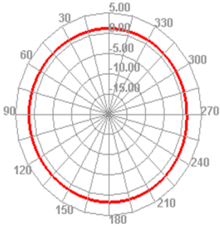
2400.000MHz E2
