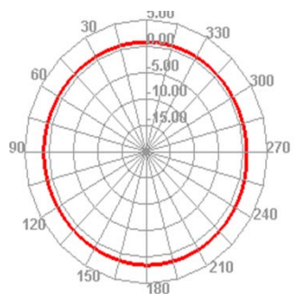
2410.000MHz E2
