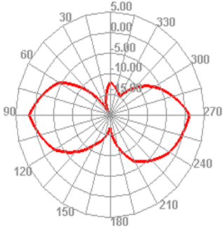
2410.000MHz H
