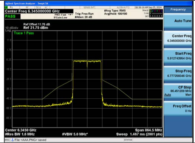
802.11be EHT160M Ch.79(6345 MHz) 2x996 Tones 68 RU
