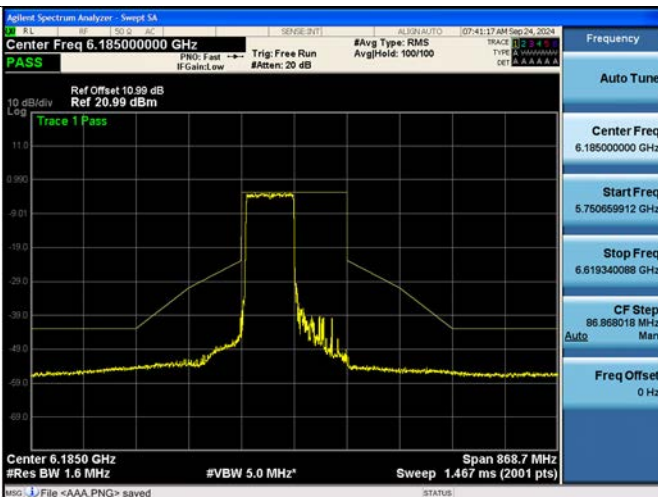
802.11be EHT160M Ch.47(6185 MHz) 996 Tones 67 RU
