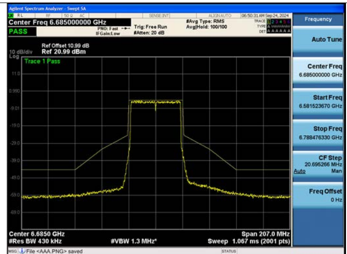
802.11be EHT40M Ch.147(6685 MHz) SU
