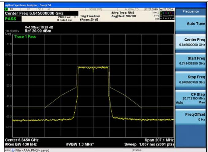
802.11be EHT40M Ch.179(6845 MHz) SU
