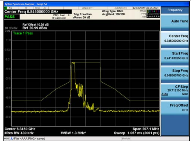
802.11be EHT40M Ch.179(6845 MHz) 242 Tones 61 RU
