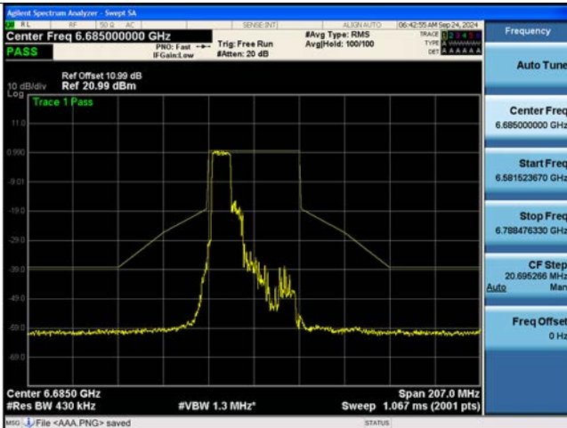
802.11be EHT40M Ch.147(6685 MHz) 484 Tones 65 RU
