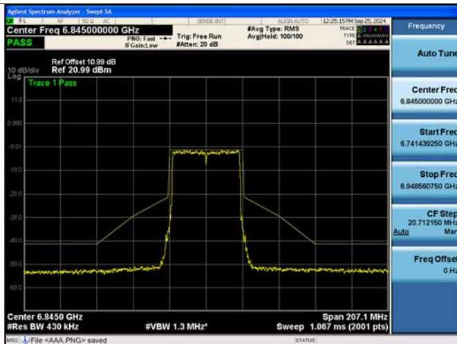
802.11be EHT40M Ch.179(6845 MHz) 484 Tones 65 RU
