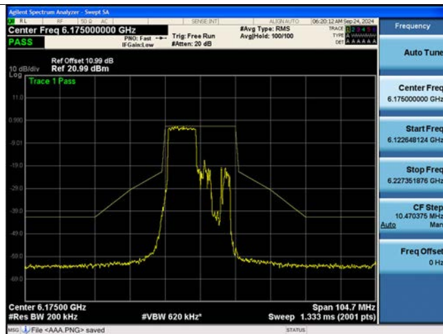
802.11be EHT20M Ch.45(6175 MHz) SU
