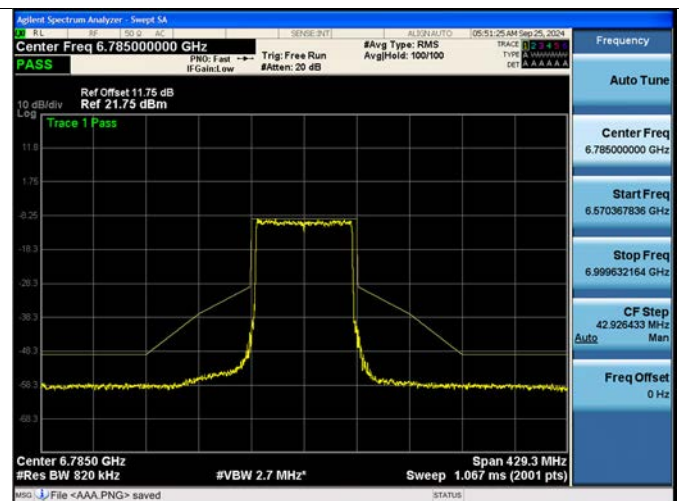
802.11be EHT80M Ch.167(6785 MHz) 996 Tones 67 RU
