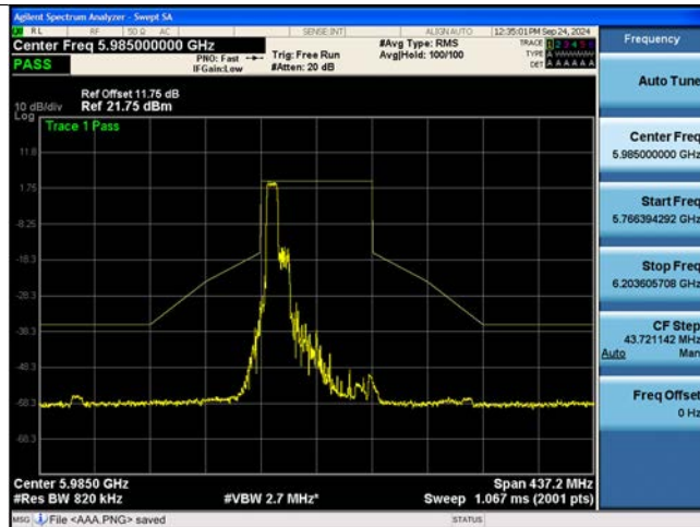
802.11be EHT80M Ch.7(5985 MHz) 484 Tones 65 RU
