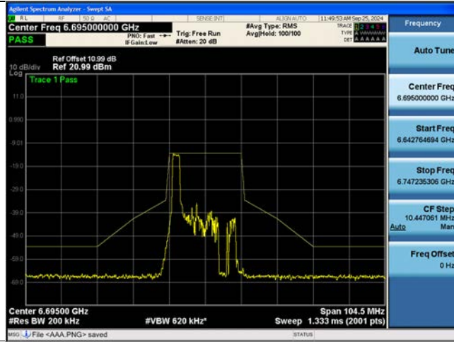
802.11be EHT20M Ch.149(6695 MHz) 106 Tones 53 RU
