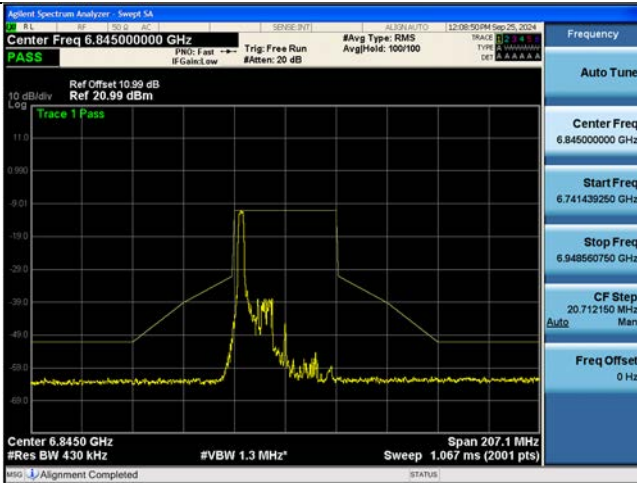
802.11be EHT40M Ch.179(6845 MHz) 106 Tones 53 RU
