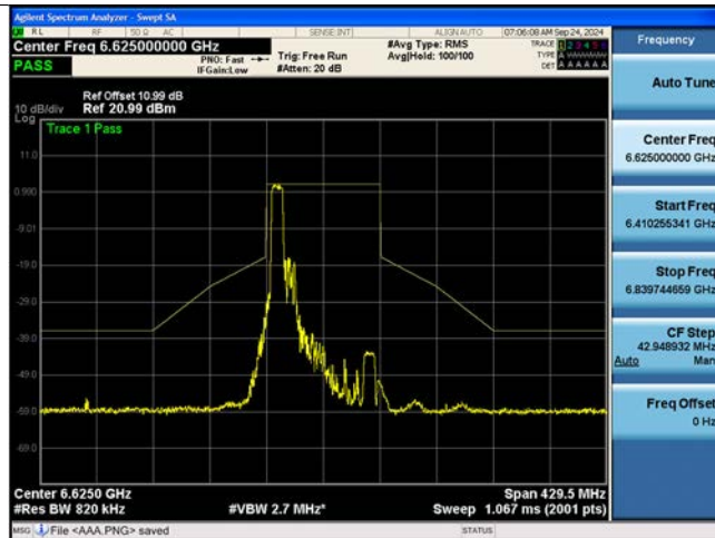
802.11be EHT80M Ch.135(6625 MHz) 484 Tones 65 RU
