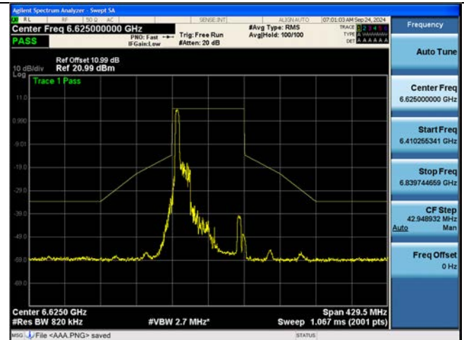
802.11be EHT80M Ch.135(6625 MHz) 242 Tones 61 RU
