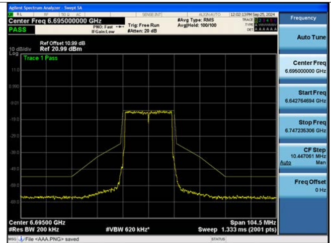
802.11be EHT20M Ch.149(6695 MHz) 242 Tones 61 RU
