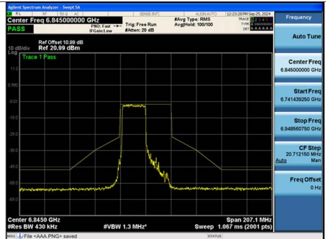
802.11be EHT40M Ch.179(6845 MHz) SU
