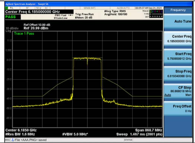
802.11be EHT160M Ch.47(6185 MHz) 2x996 Tones 68 RU
