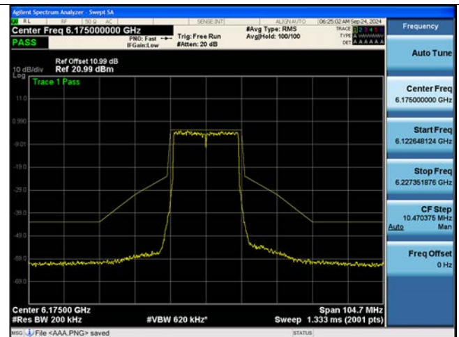
802.11be EHT20M Ch.45(6175 MHz) 242 Tones 61 RU
