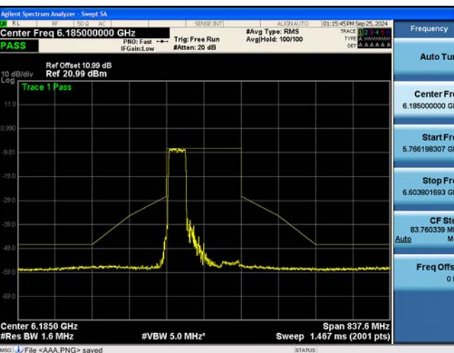
802.11be EHT160M Ch.47(6185 MHz) 484 Tones 65 RU
