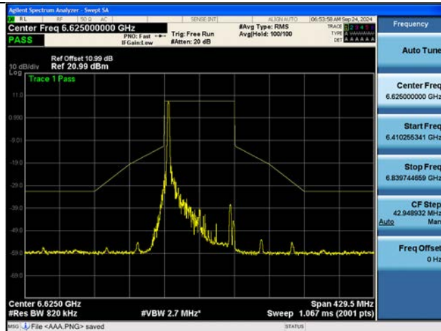
802.11be EHT80M Ch.135(6625 MHz) 106 Tones 53 RU
