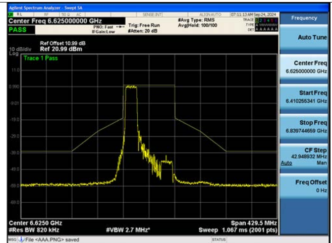
802.11be EHT80M Ch.135(6625 MHz) 996 Tones 67 RU
