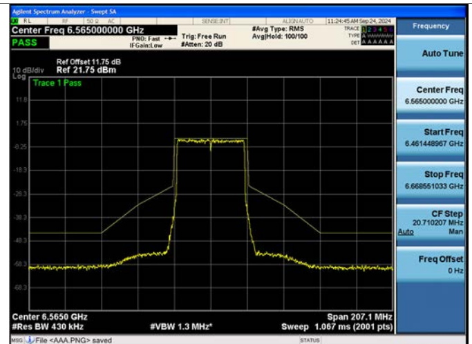
802.11be EHT40M Ch.123(6565 MHz) SU
