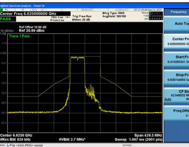
802.11be EHT80M Ch.135(6625 MHz) 484 Tones 65 RU
