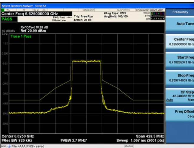
802.11be EHT80M Ch.135(6625 MHz) 996 Tones 67 RU
