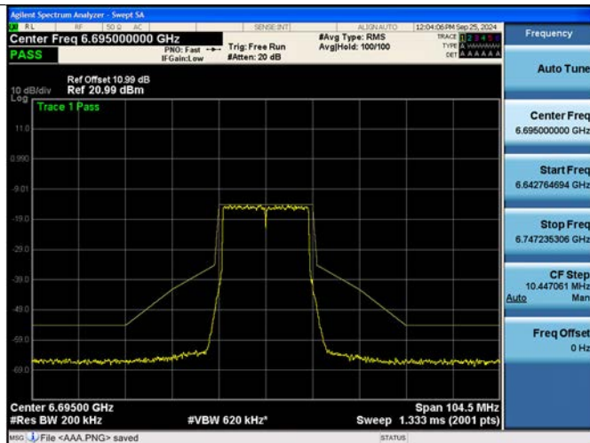
802.11be EHT20M Ch.149(6695 MHz) SU
