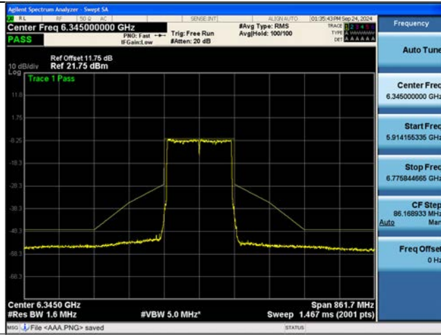
802.11be EHT160M Ch.79(6345 MHz) SU
