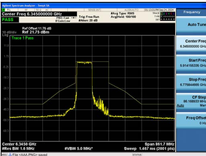
802.11be EHT160M Ch.79(6345 MHz) 996 Tones 67 RU
