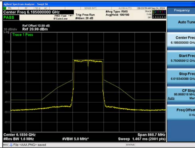
802.11be EHT160M Ch.47(6185 MHz) SU
