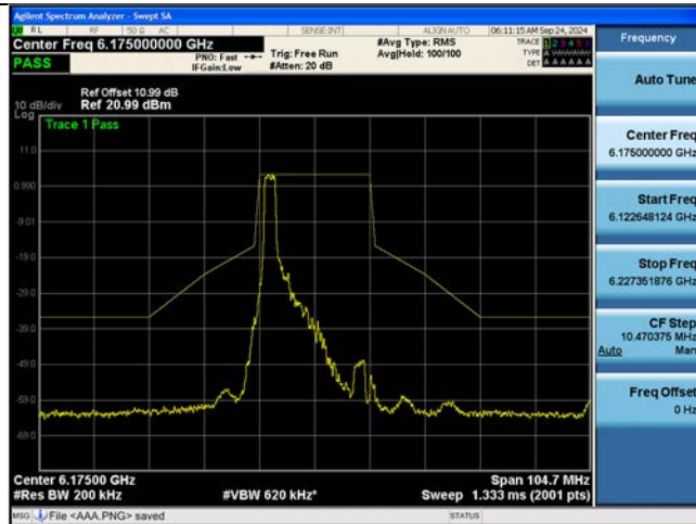
802.11be EHT20M Ch.45(6175 MHz) 106 Tones 53 RU
