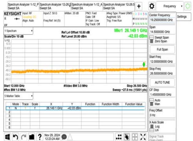
802.11ax_20MHz_2472MHz_RU52_40
