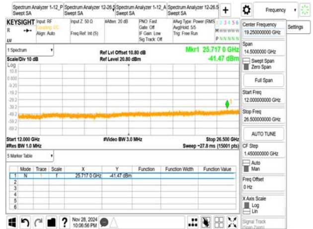
802.11ax_20MHz_2412MHz_RU242
