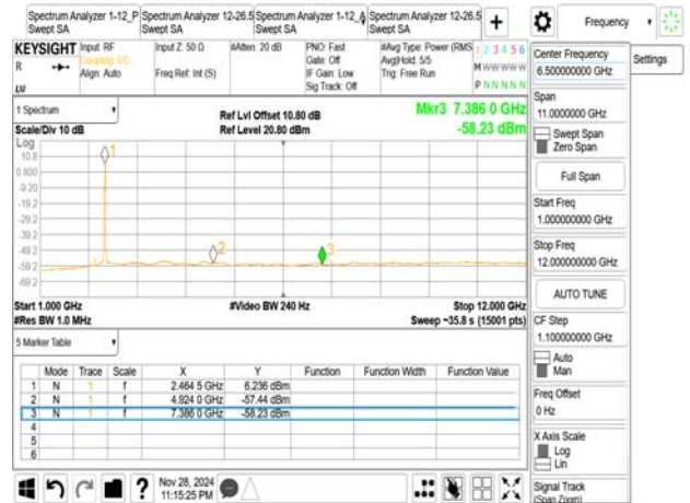
802.11ax_20MHz_2462MHz_RU242
