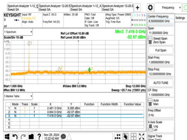
802.11ax_20MHz_2472MHz_RU52_40
