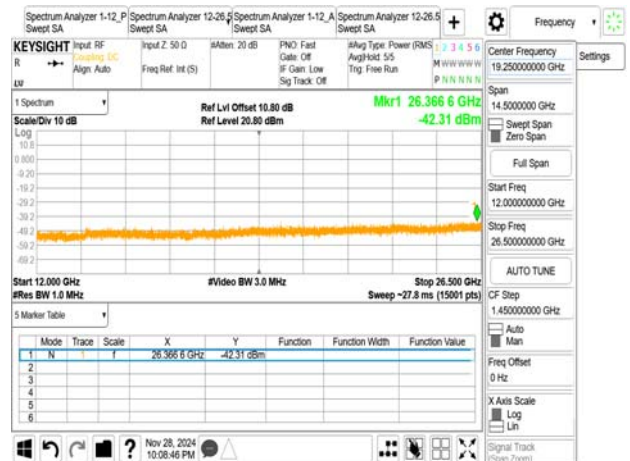
802.11ax_20MHz_2412MHz_RU26_0
