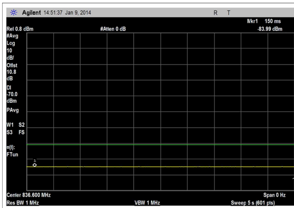
UL_824-849MHz_single_-70dBm
