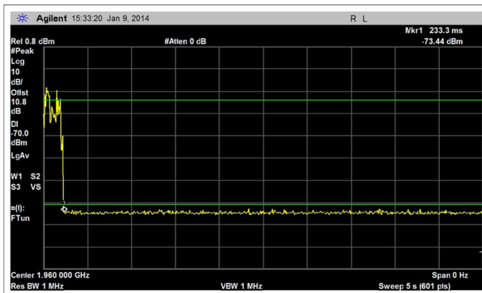
DL_1930-1995MHz_single
