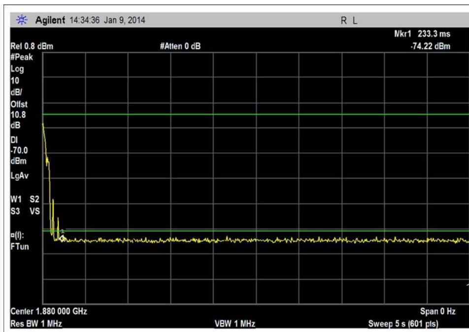
UL_1850-1915_single
