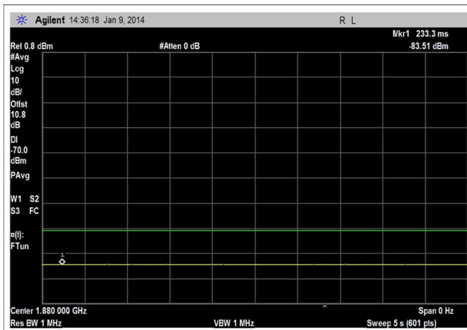
UL_1850-1915_single_-70dBm
