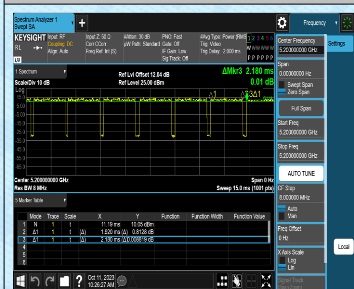
NTNV-11AC20MIMO-Ant1-5200
