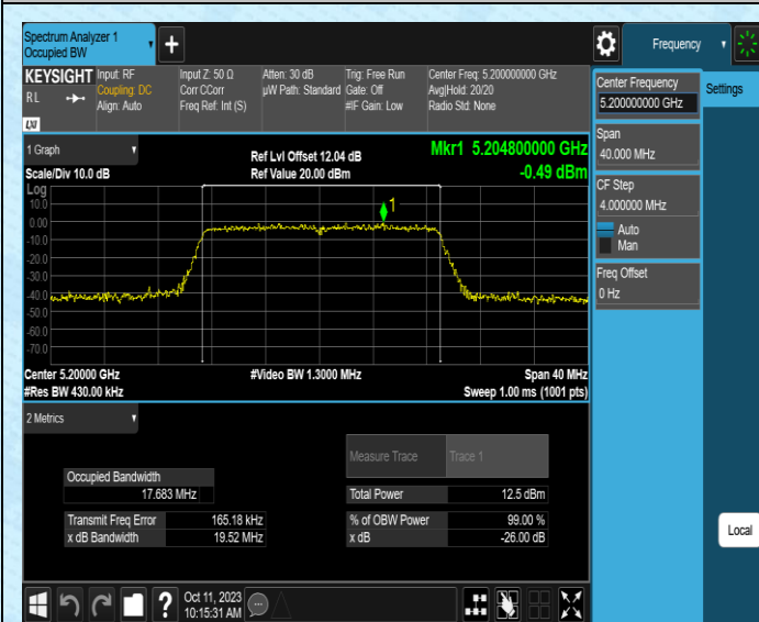
11N20MIMO-Ant1-5200
