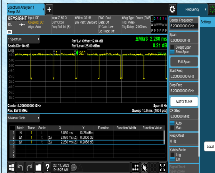
NTNV-11A-Ant1-5200
