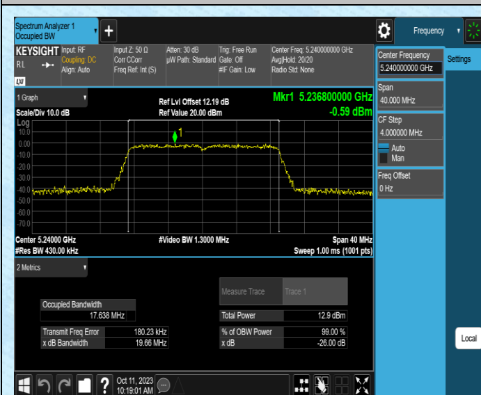
11N20MIMO-Ant1-5240
