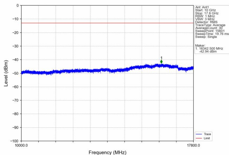
Band66 10MHz QPSK HCH 1775MHz RB 1 49 NTNV
