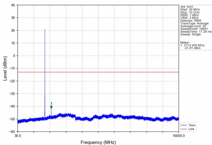
Band66 5MHz 16QAM LCH 1712.5MHz RB 1 0 NTV
