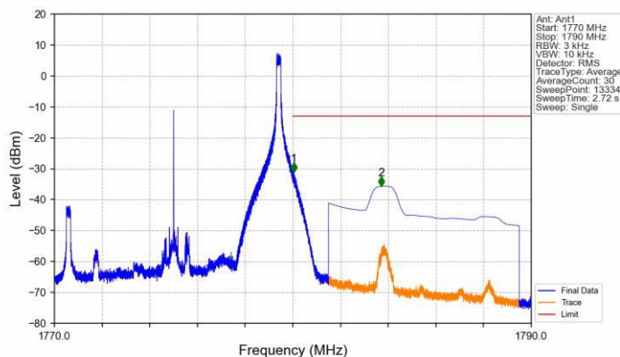
Band66 10MHz QPSK HCH 1775MHz RB 1 49 NTNV
