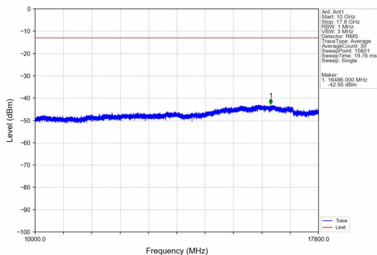
Band66 5MHz QPSK HCH 1777.5MHz RB 1 24 NTV
