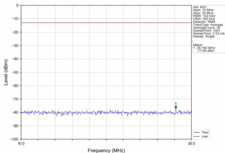
Band66 5MHz 16QAM LCH 1712.5MHz RB 1 0 NTV
