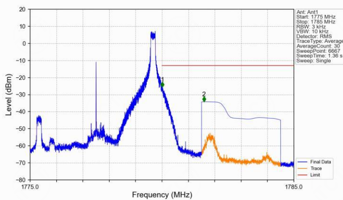
Band66 5MHz QPSK HCH 1777.5MHz RB 1 24 NTV
