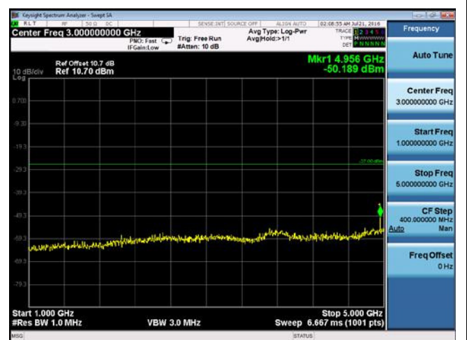
CUE-802.11n-40-5230M -chain4(1GHz-5GHz)
