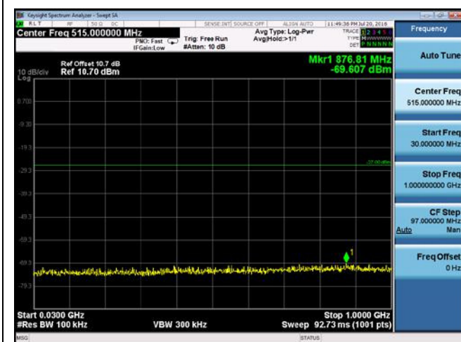
CUE-802.11n-20-5785M-chain1(30MHz-1GHz)
