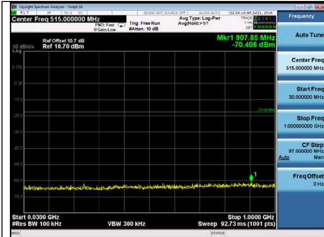
CUE-802.11n-20-5745M-chain4(30MHz-1GHz)
