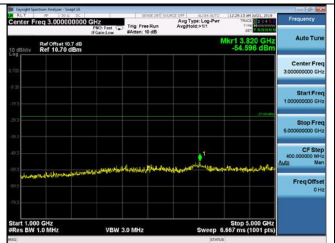
CUE-802.11n-20-5785M -chain2(1GHz-5GHz)
