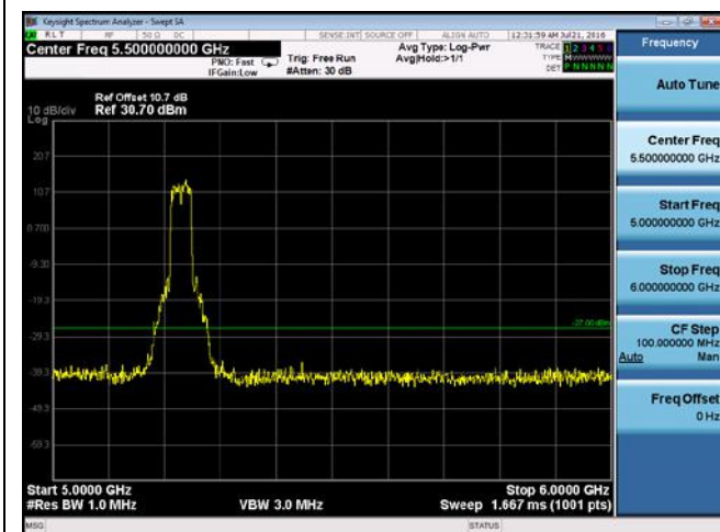
CUE-802.11n-40-5230M -chain2(5GHz-6GHz)
