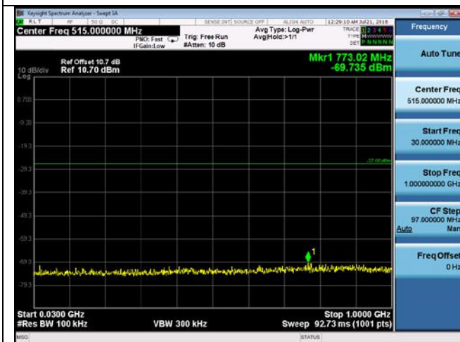
CUE-802.11n-20-5785M -chain2(30MHz-1GHz)
