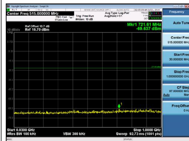
CUE-802.11n-20-5785M -chain4(30MHz-1GHz)
