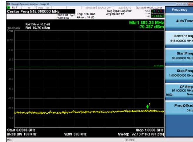
CUE-802.11n-40-5755M-chain4(30MHz-1GHz)
