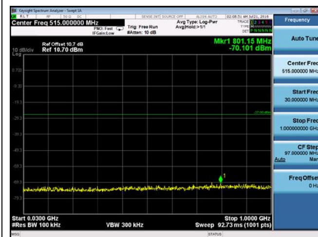
CUE-802.11n-40-5230M -chain4(30MHz-1GHz)
