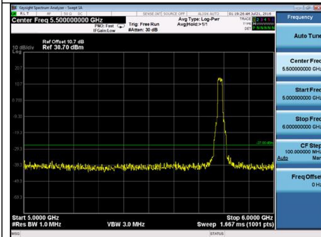
CUE-802.11n-20-5785M -chain3(5GHz-6GHz)
