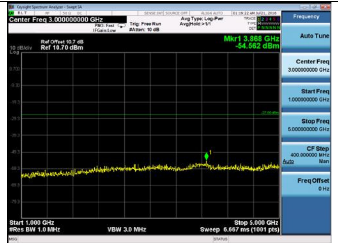
CUE-802.11n-20-5785M -chain3(1GHz-5GHz)
