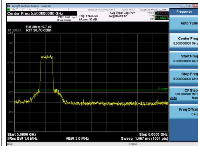
CUE-802.11ac-80-5210M -chain 4(5GHz-6GHz)
