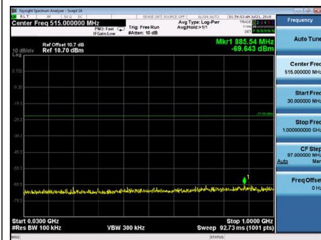
CUE-802.11a-5785M-chain4(30MHz-1GHz)
