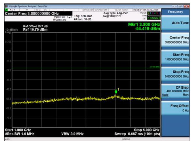
CUE-802.11n-20-5785M -chain4(1GHz-5GHz)
