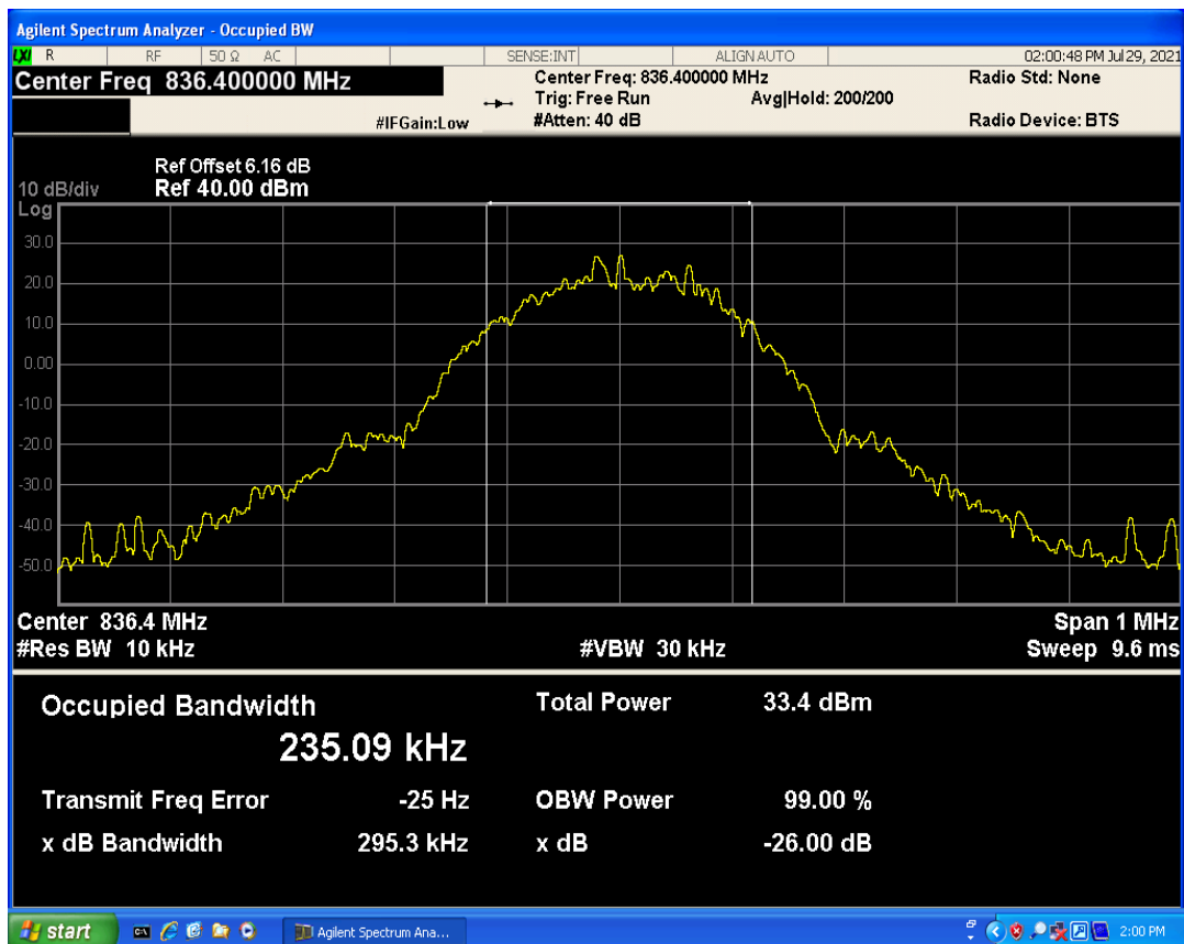
17 Band edge
