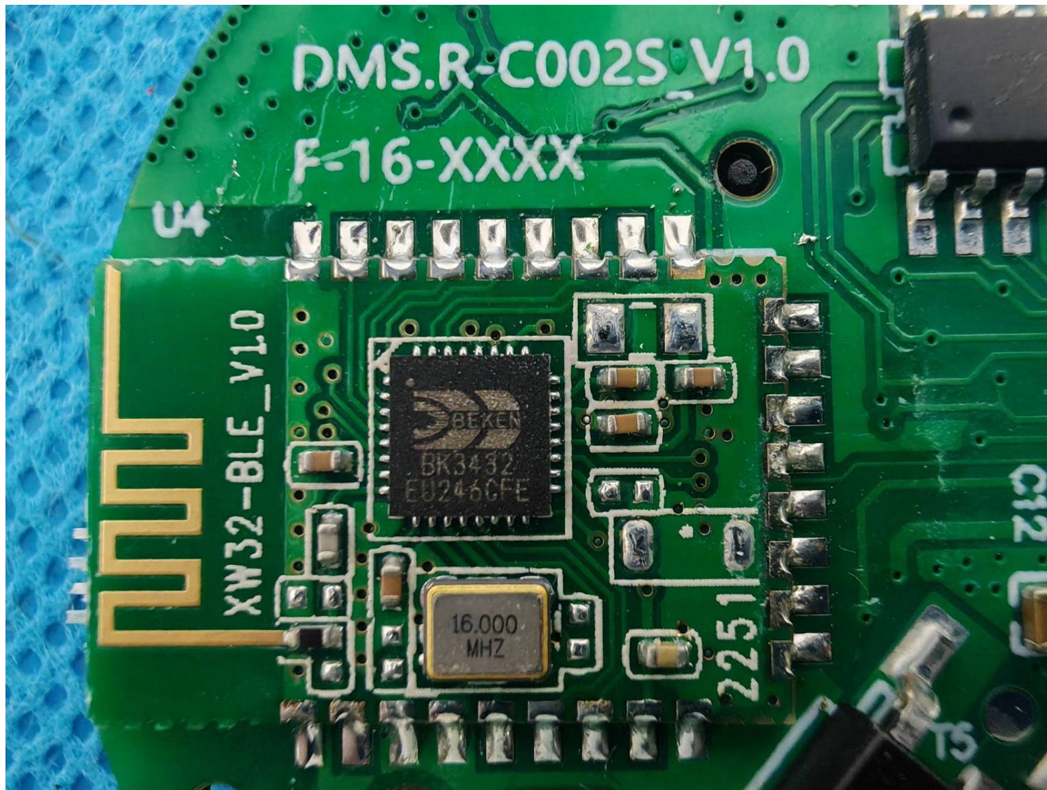
RF Module
