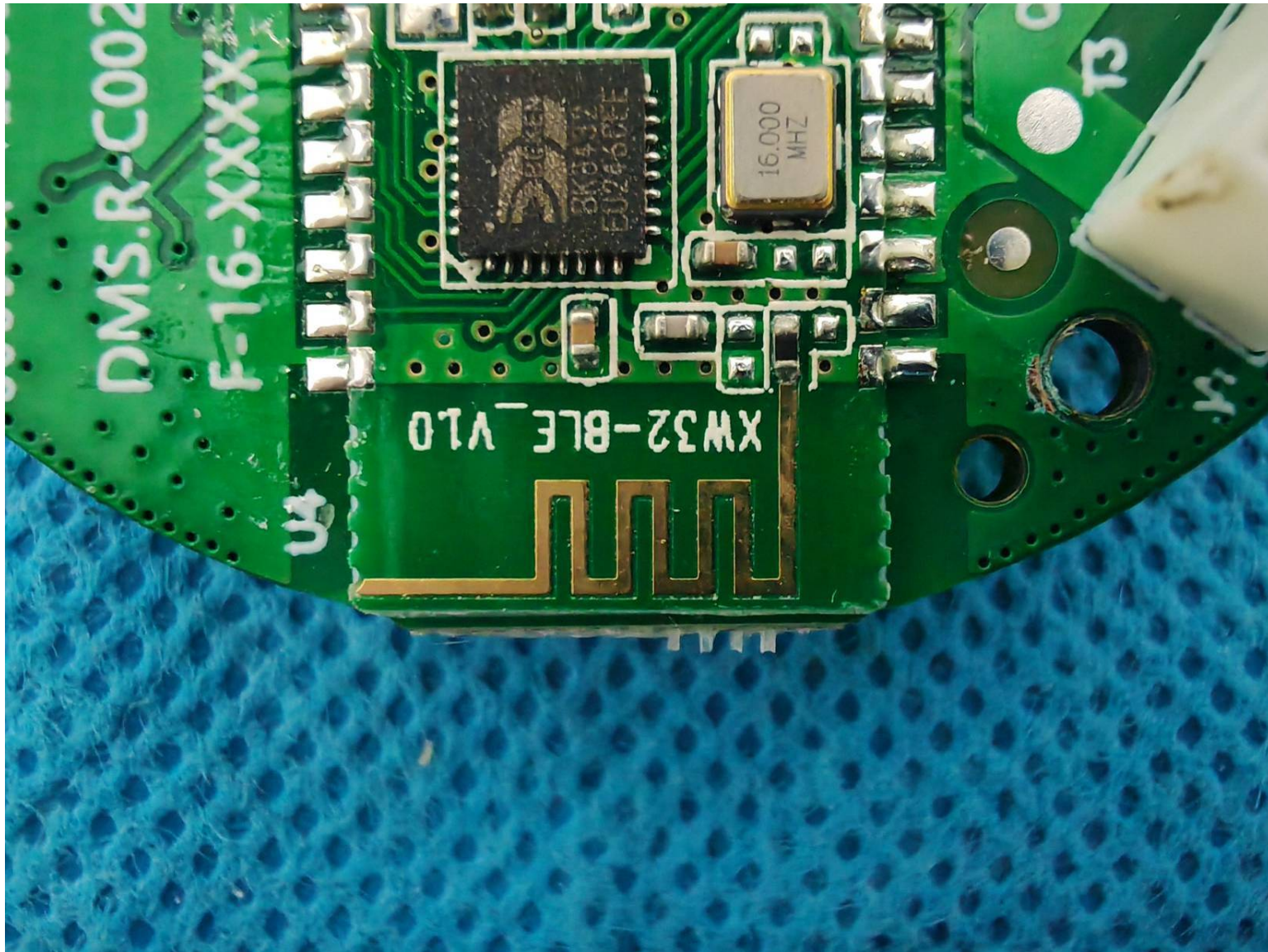
Antenna
