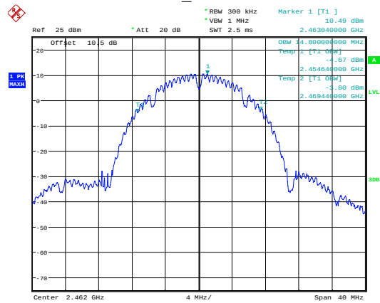
b_2462MHz
