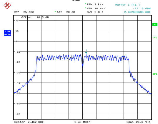
g_2462MHz
