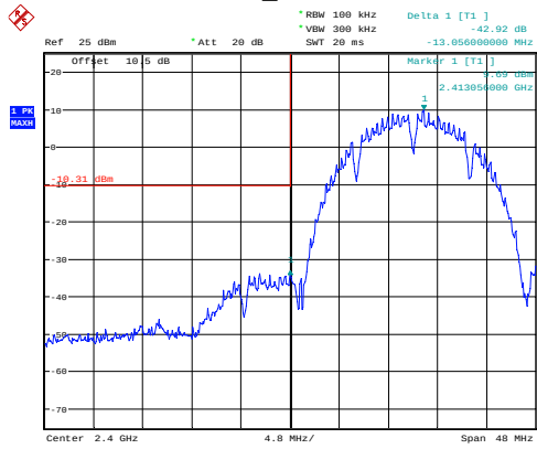
b_2412MHz
