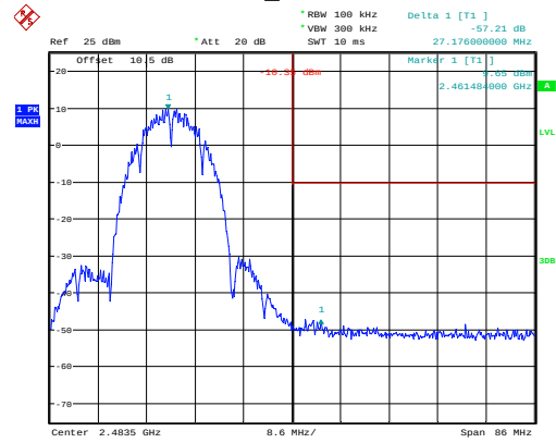
b_2462MHz
