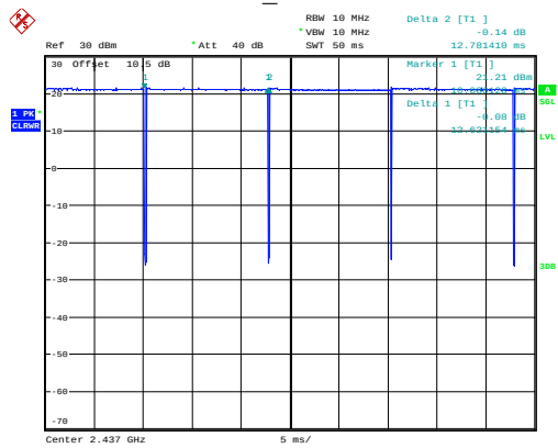
b_2437MHz
