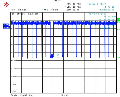
g_2437MHz
