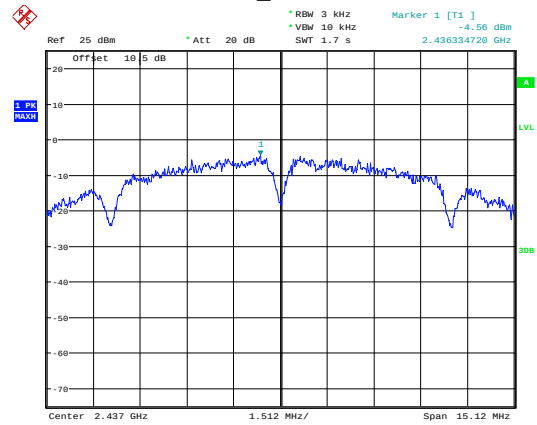
b_2437MHz
