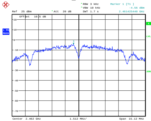
b_2462MHz
