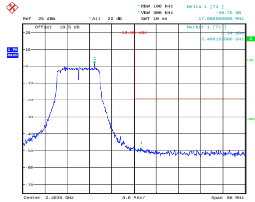
g_2462MHz
