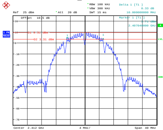
b_2412MHz
