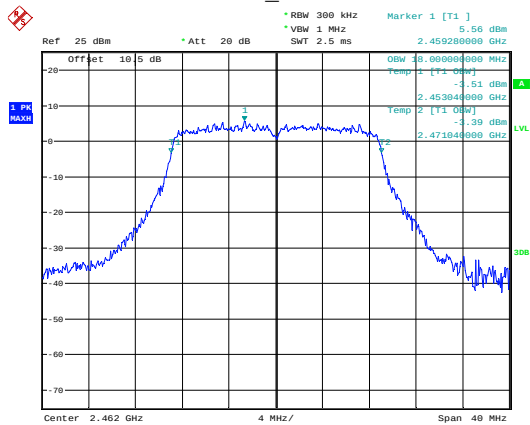
n20_2462MHz
