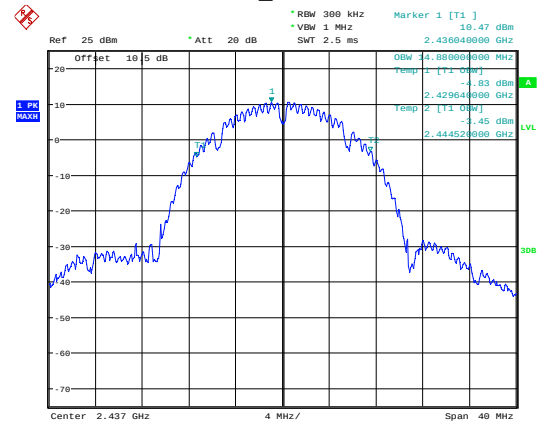
b_2437MHz
