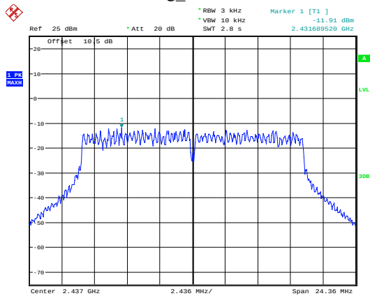
g_2437MHz
