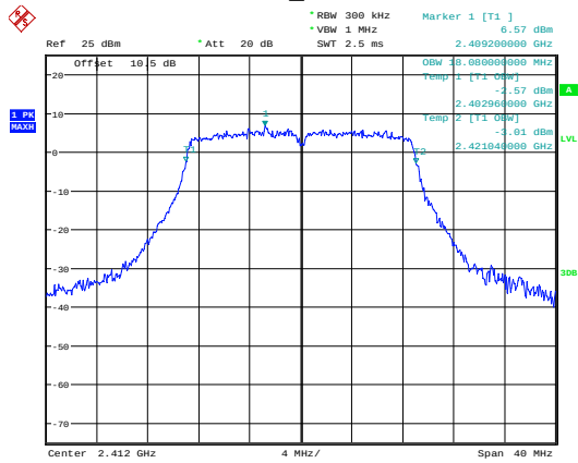
n20_2412MHz
