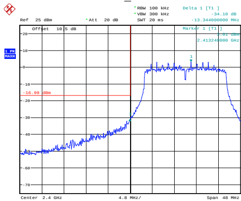
n20_2412MHz
