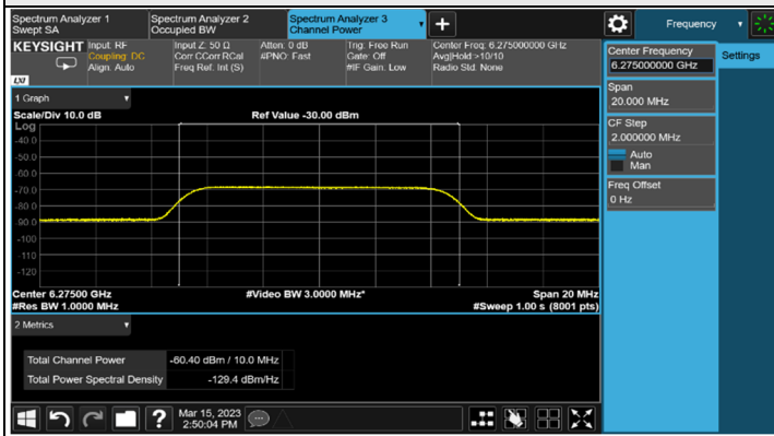
802.11be (HE20) / CH65
