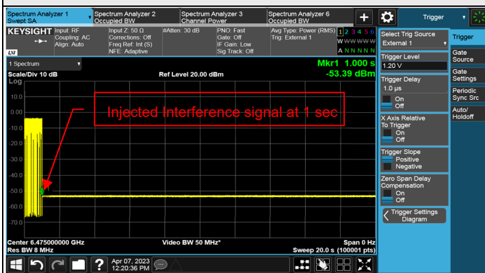
802.11be (HE20) / CH105
