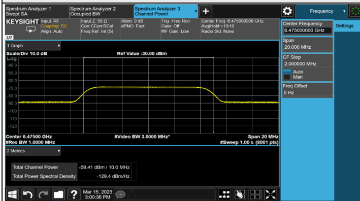
802.11be (HE20) / CH105
