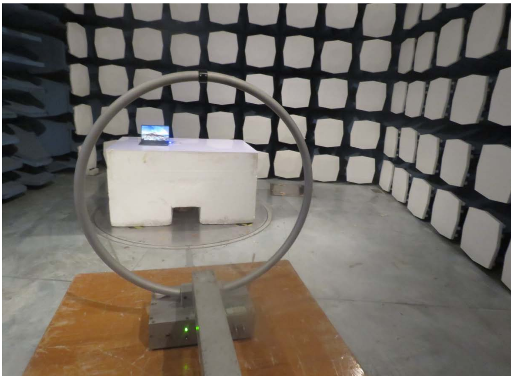
9kHz-30MHz
