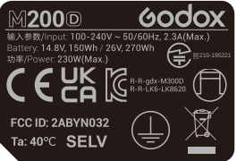
707-M200D0-02右侧贴纸 707-M200D0-02 right side sticker
