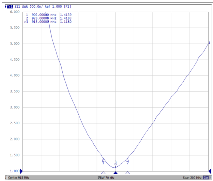
V.S.W.R
