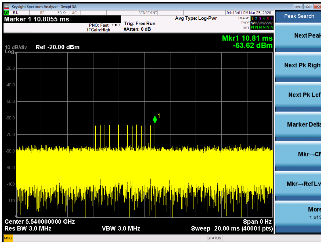
Radarsignal 4
