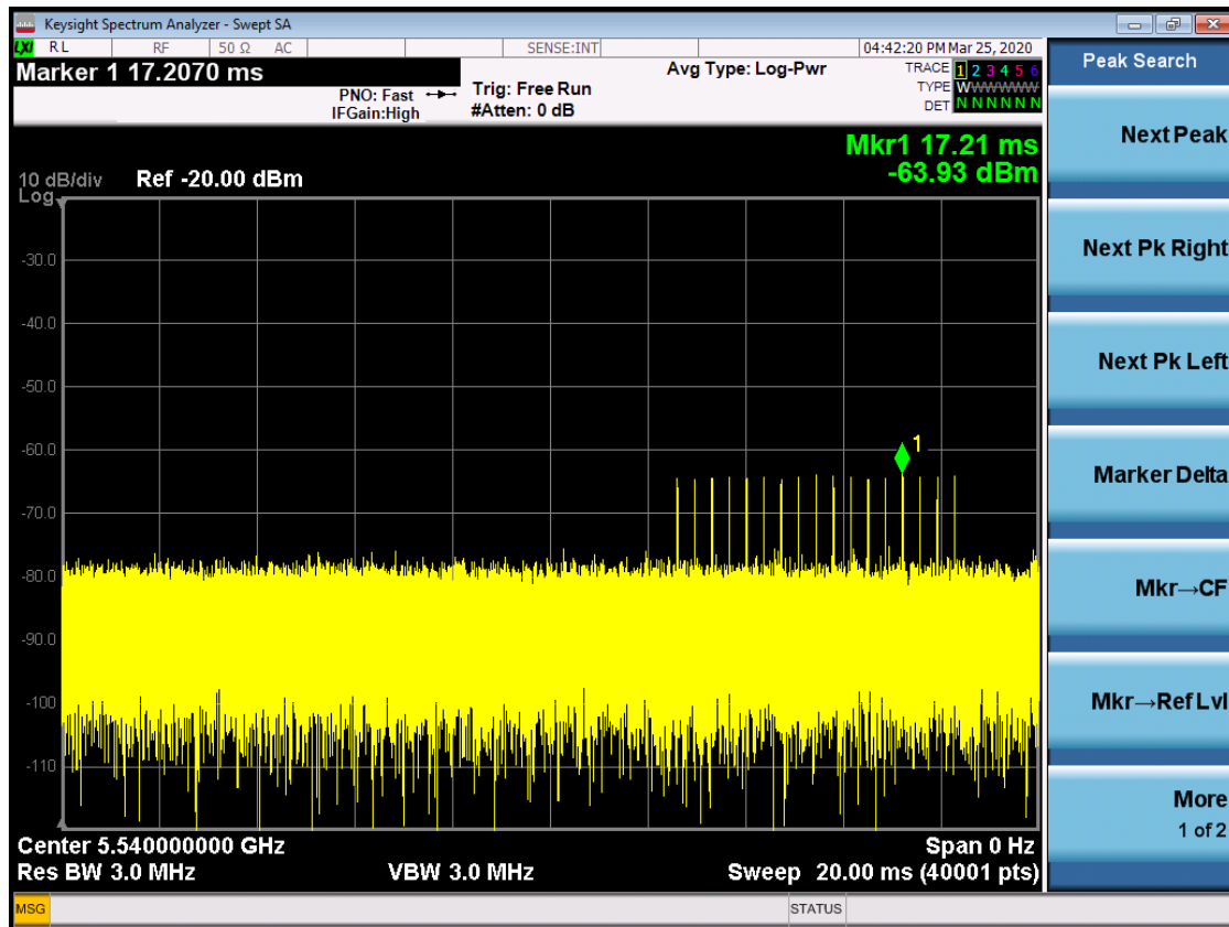
Radarsignal 4
