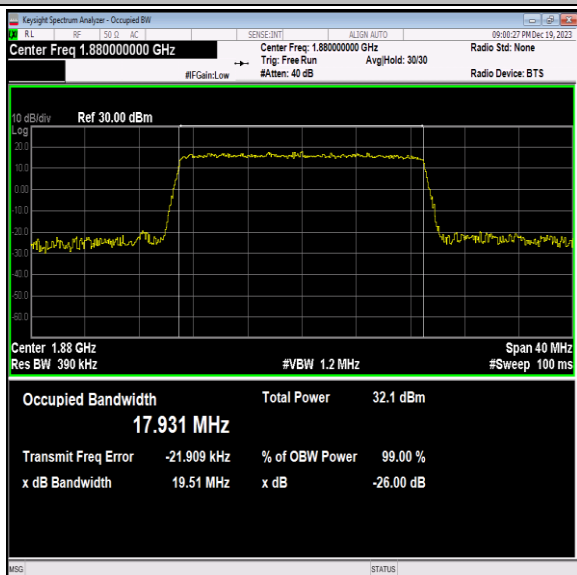
Band2-20MHz-QPSK-18900-100RB#0-PASS
