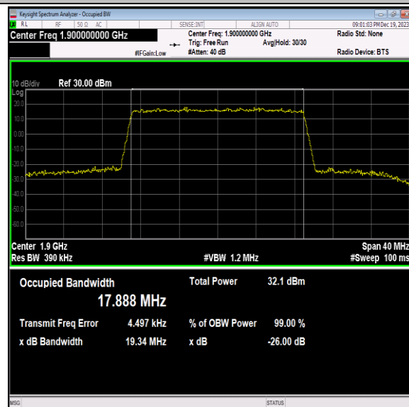
Band2-20MHz-QPSK-19100-100RB#0-PASS
