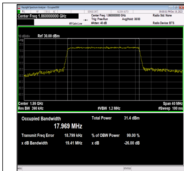
Band2-20MHz-16QAM-18700-100RB#0-PASS
