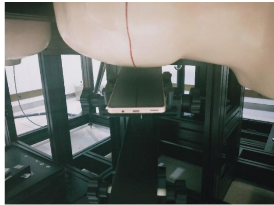
Right Tilt
