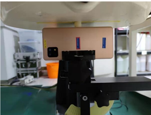
Left(10mm)
