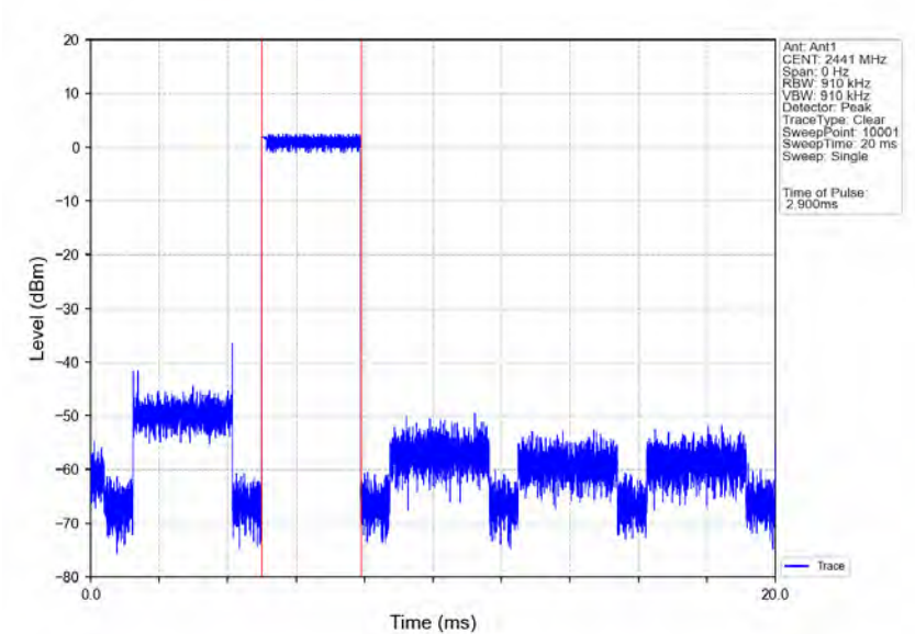
8DPSK_3DH5_HOPP_Ant1_NTNV
