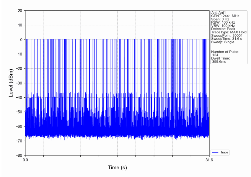
Pi/4DQPSK_2DH5_HOPP_Ant1_NTNV
