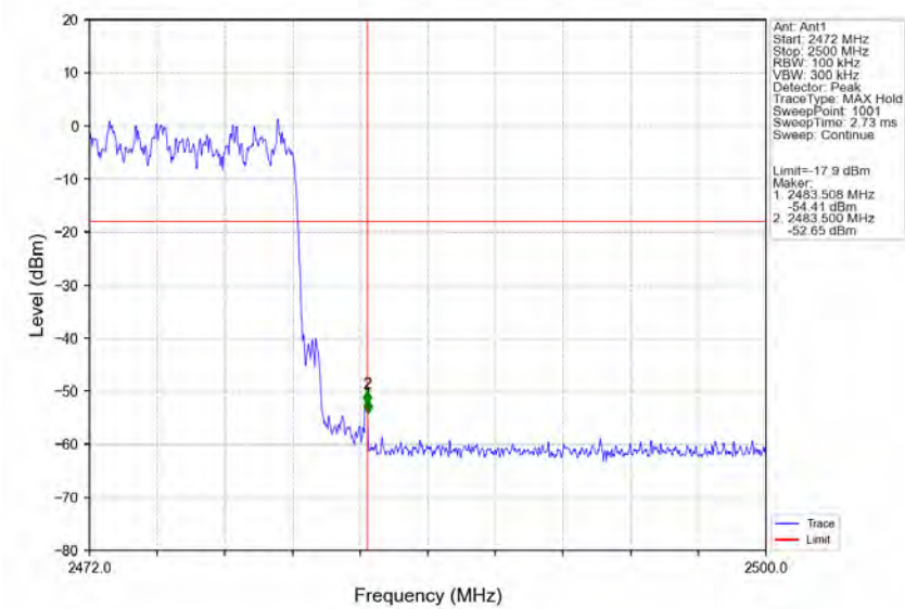
8DPSK_3DH5_HOPP_Ant1_NTNV
