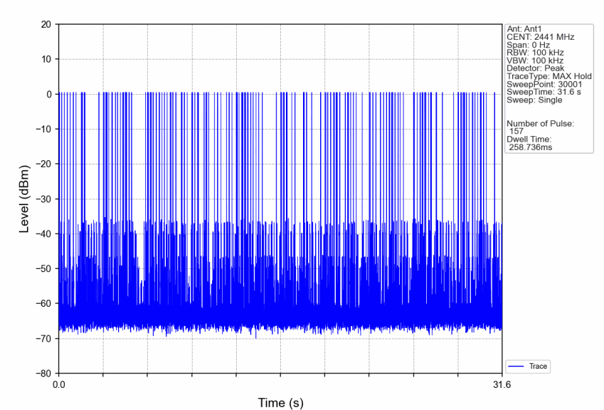
Pi/4DQPSK_2DH3_HOPP_Ant1_NTNV
