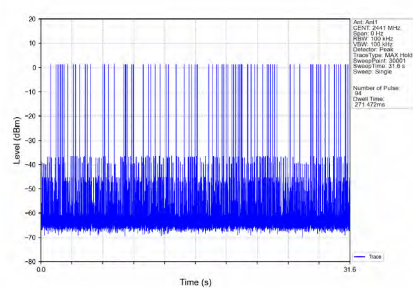
GFSK_DH5_HOPP_Ant1_NTNV
