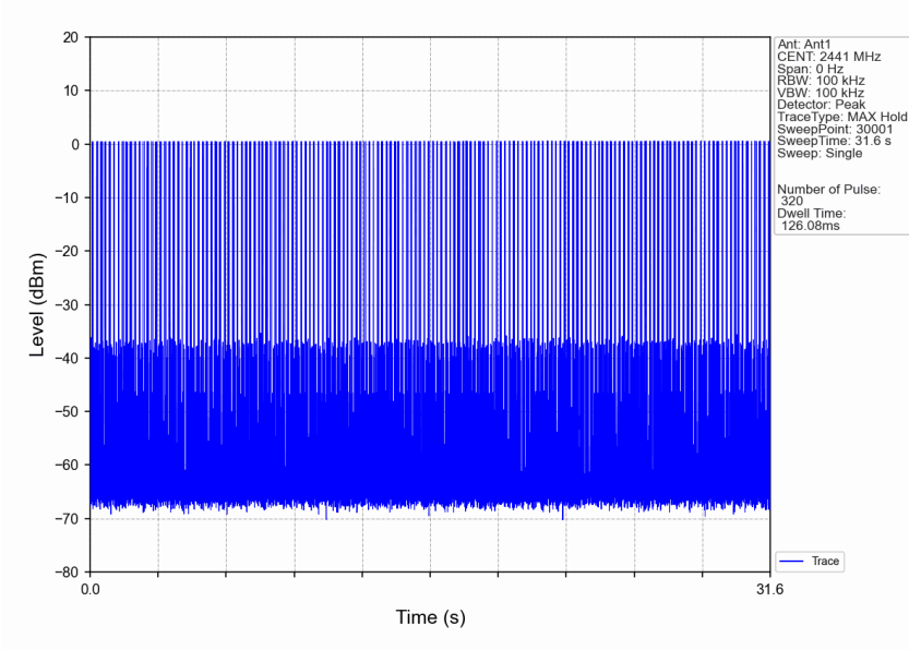
Pi/4DQPSK_2DH1_HOPP_Ant1_NTNV
