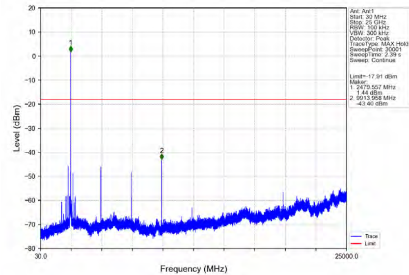
GFSK_DH5_HOPP_Ant1_NTNV
