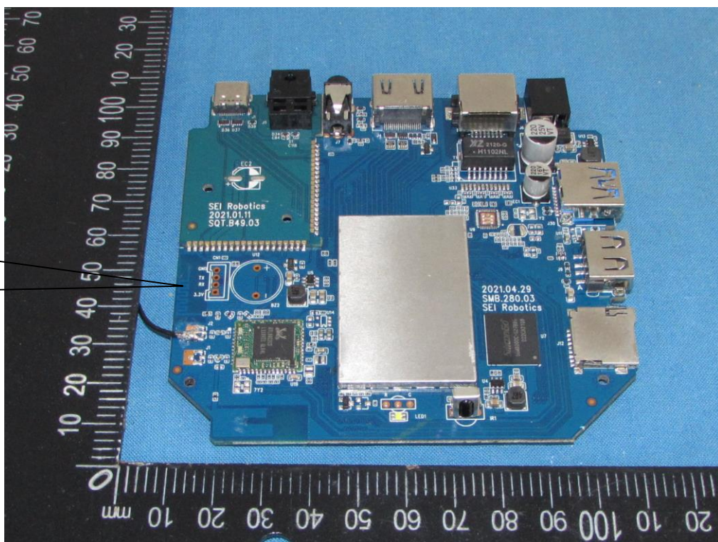
Bluetooth Antenna [Antenna 3]
