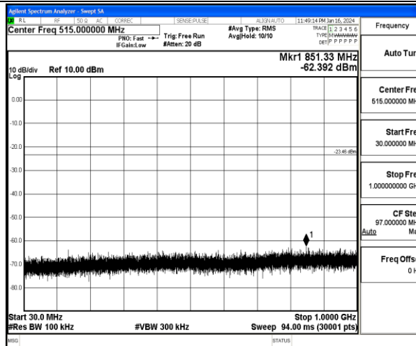
11G-Ant1-2412-30~1000-PASS
