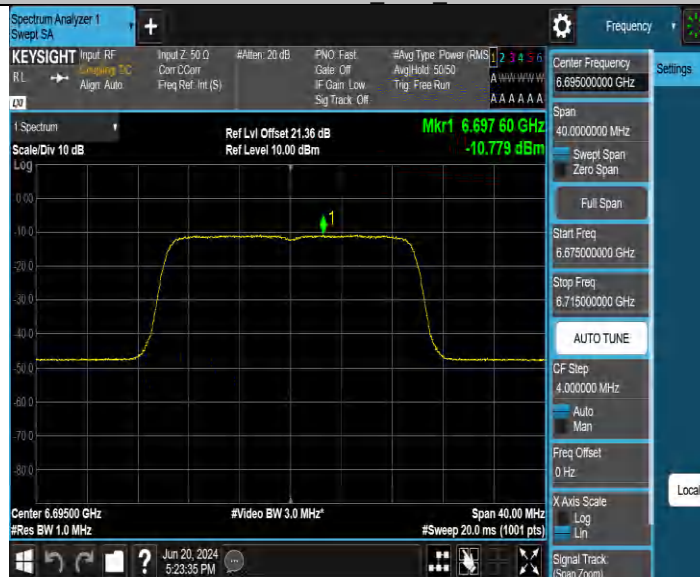
11BE20MIMO_Ant3_6695
