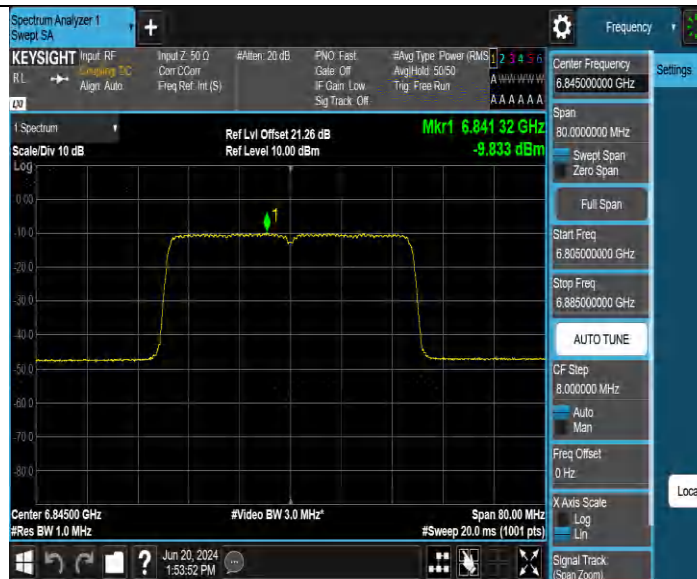
11AX40MIMO_Ant4_6845
