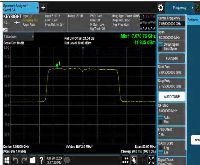
11AX40MIMO_Ant3_7085
