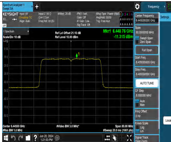
11AX40MIMO_Ant3_6445
