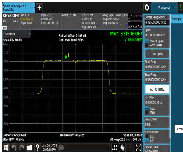
11AX40MIMO_Ant2_6925
