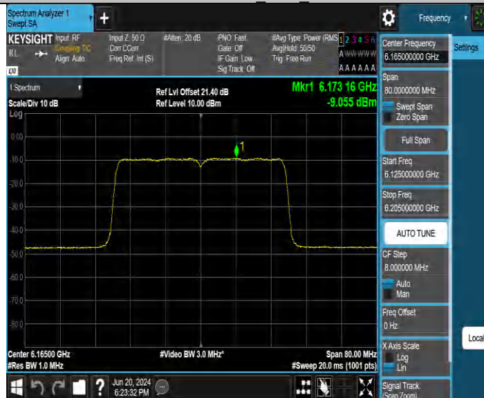
11BE40MIMO_Ant2 6165
