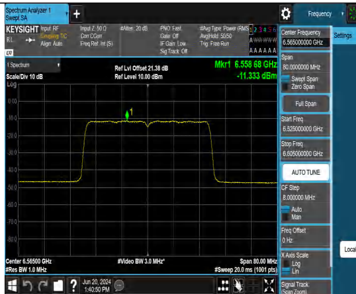
11AX40MIMO_Ant3_6565
