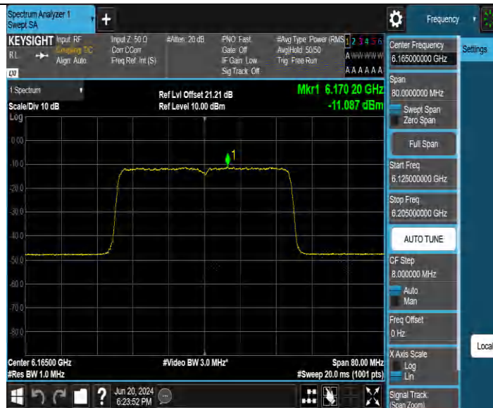
11BE40MIMO_Ant3_6165
