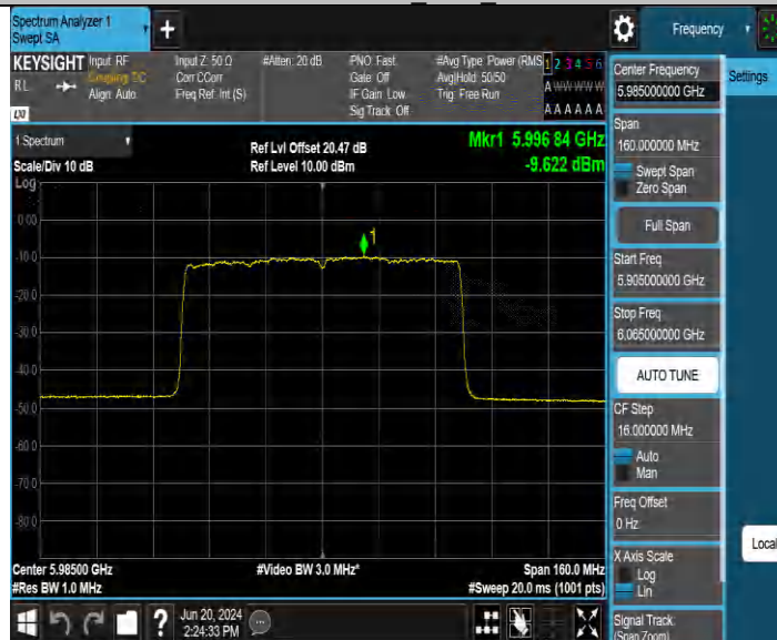
11AX80MIMO_Ant4_5985
