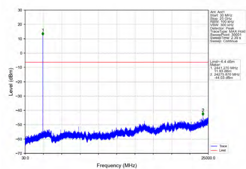
Pi/4DQPSK 2DH5 MCH 2441MHz Ant1 NTN
