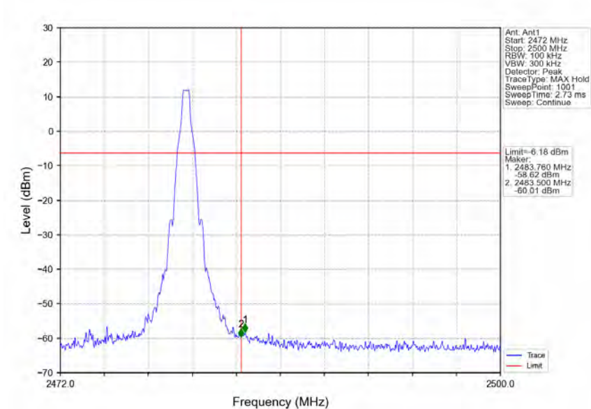
GFSK DH5 HCH 2480MHz Ant1 NTNV
