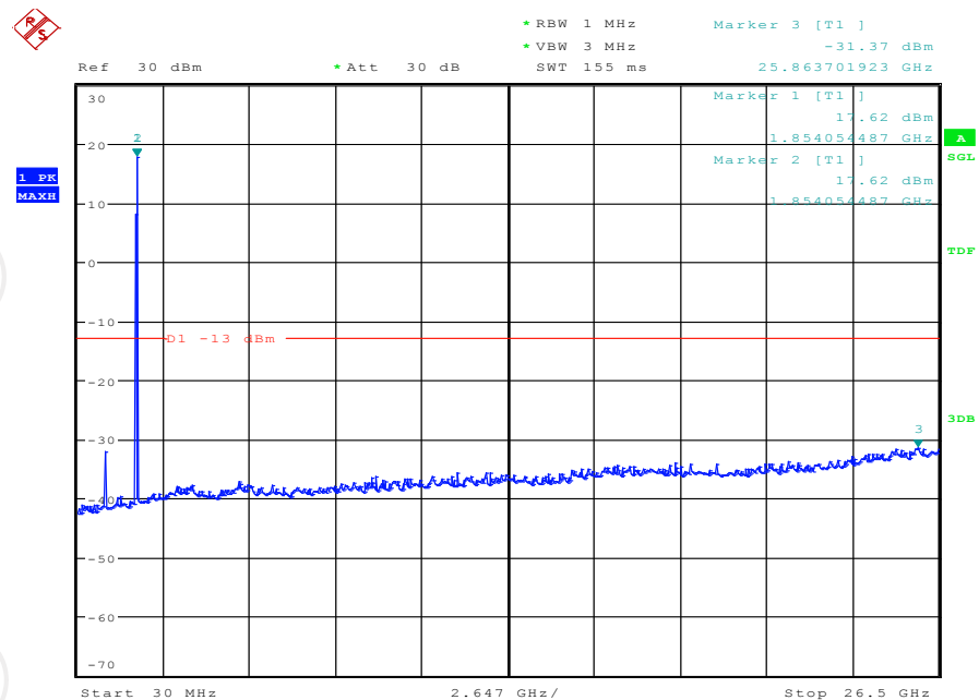
BW1.4MHz-1850.7MHz,QPSK-6RB_LOW@Pass
