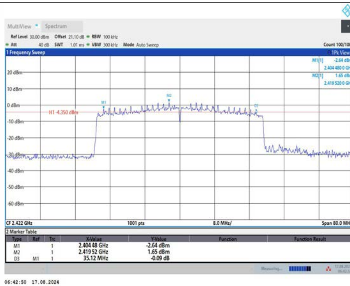
11BE40MIMO_Ant2_2422
