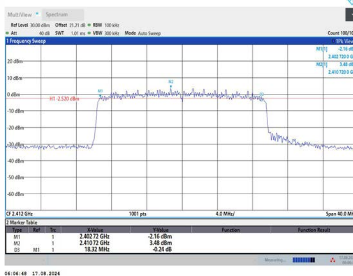
11AX20MIMO_Ant1_2412
