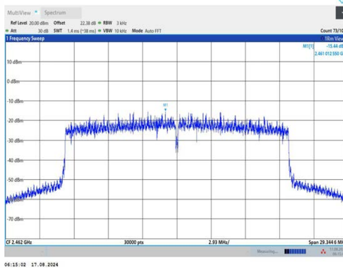
11AX20MIMO_Ant2_2462
