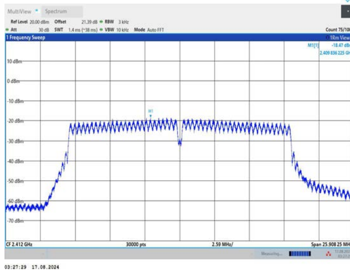
11G_Ant2_2412
