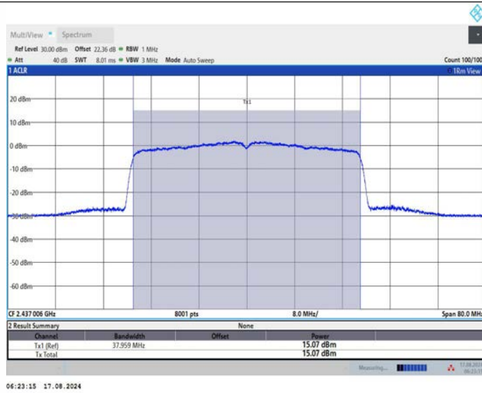
11AX40MIMO_Ant2_2437
