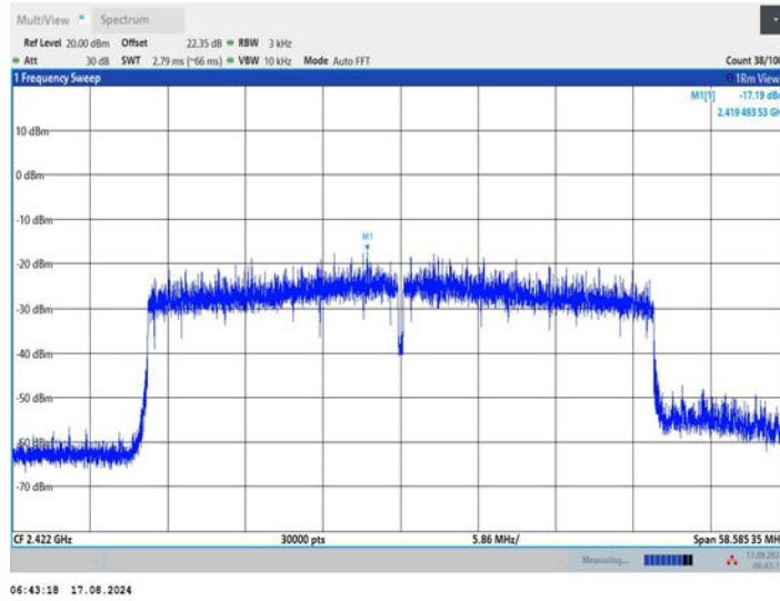
11BE40MIMO_Ant2_2422
