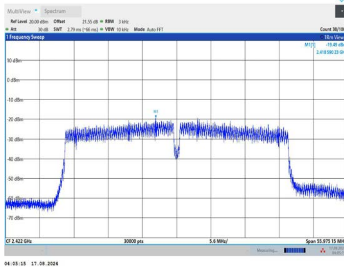
11N40MIMO_Ant2_2422
