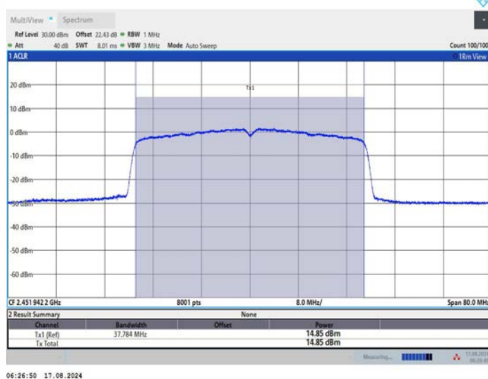
11AX40MIMO_Ant1_2452
