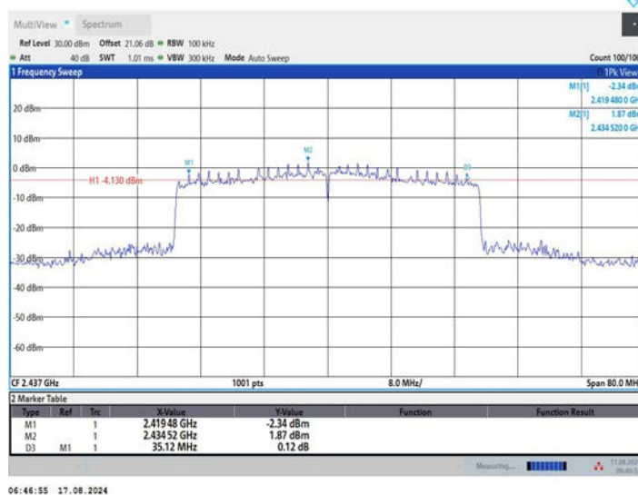
11BE40MIMO_Ant1_2437
