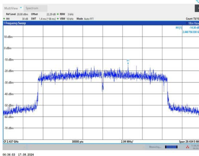
11BE20MIMO_Ant2_2437
