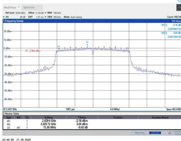
11G_Ant2_2437
