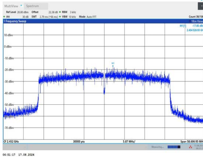
11BE40MIMO_Ant2_2452
