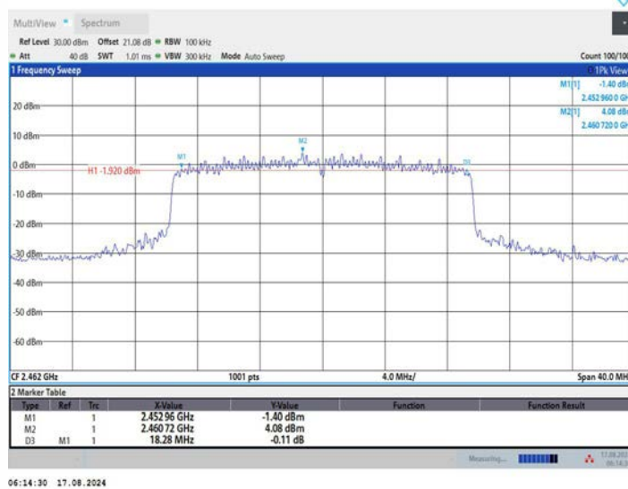
11AX20MIMO_Ant2_2462
