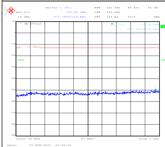
Band2-1.4MHz-QPSK-19193:30~1000MHz
