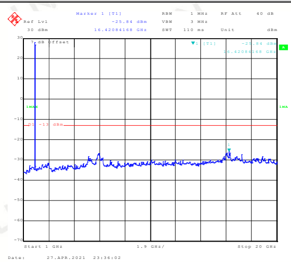
Band2-1.4MHz-QPSK-19193:1000~20000MHz
