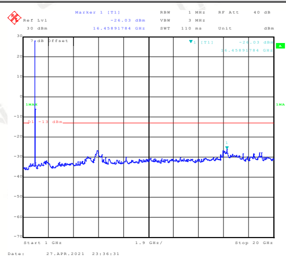
Band2-1.4MHz-QPSK-19193:1000~20000MHz
