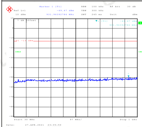
Band2-1.4MHz-QPSK-19193:30~1000MHz
