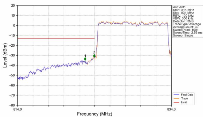
Band26b 10MHz QPSK LCH 829MHz RB 50 0 NTNV
