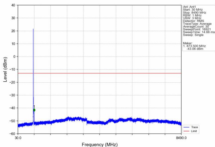
Band26b 10MHz QPSK LCH 829MHz RB 50 0 NTNV
