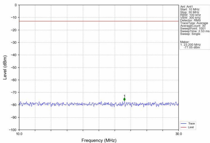
Band26b 10MHz QPSK LCH 829MHz RB 1 0 NTNV
