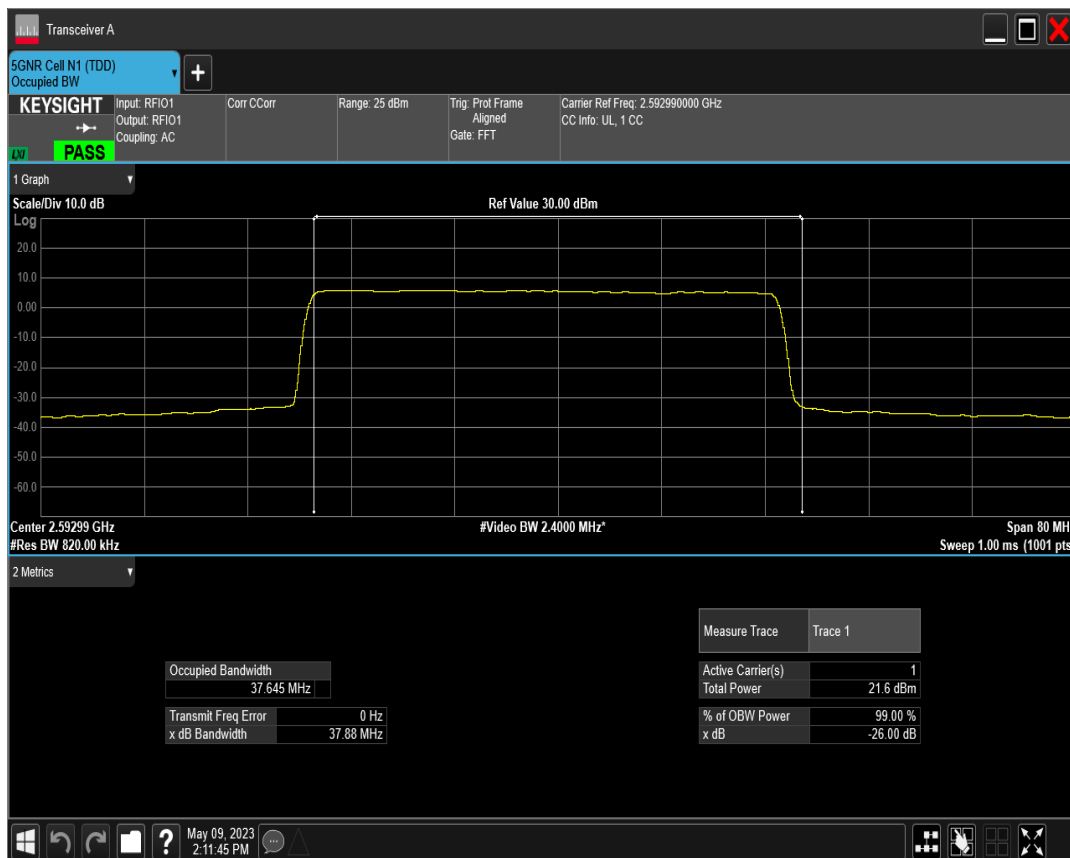
n41 SCS=30kHz CP_QPSK BW=40MHz Channel=518598 RB=106@0
