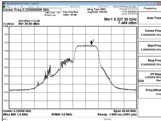
802.11ax_20MHz_RU_26_8_5320MHz-5320
