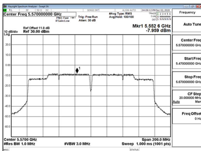
802.11ac_160MHz_5570MHz-5570
