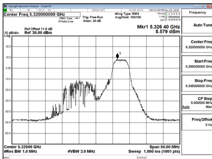
802.11ax_20MHz_RU_52_40_5320MHz-5320
