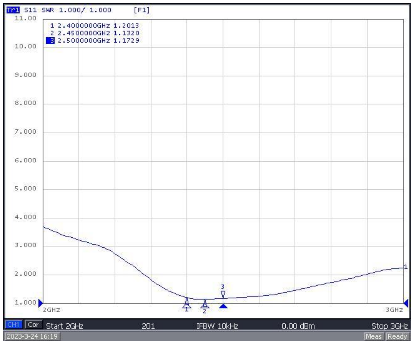
附图二：V.S.W.R
