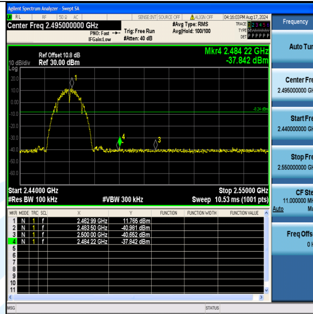
11B-Ant2-2462-PASS
