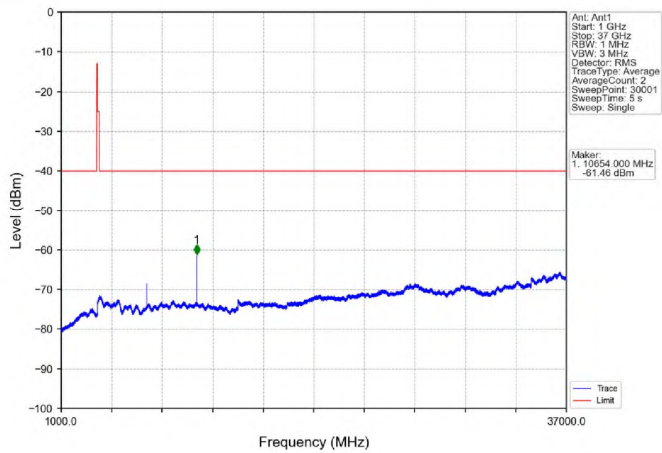
n48_30kHz_SISO_NTNV_10MHz_DFT-s-OFDM_QPSK_3555MHz_Inner_1RB_Left
