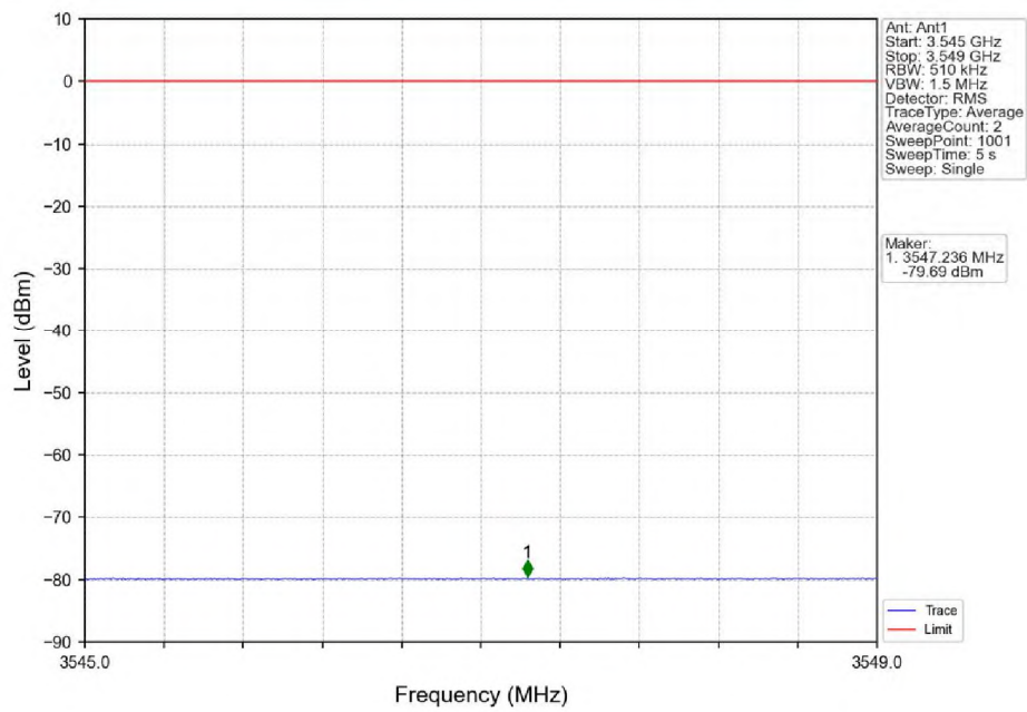
n48_30kHz_SISO_NTNV_10MHz_CP-OFDM_QPSK_3555MHz_Edge_1RB_Left
