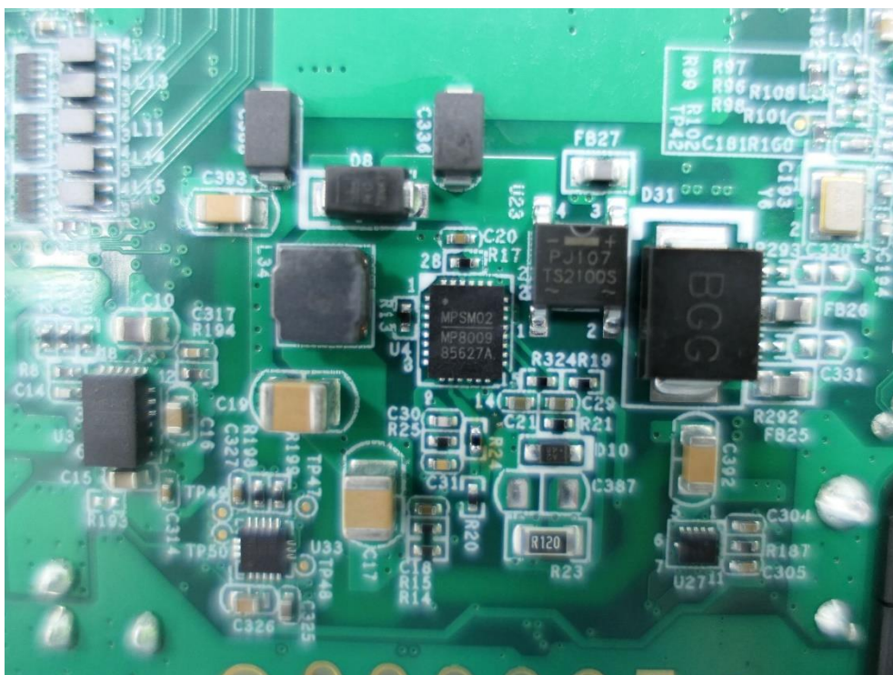
(24) EUT Photo
