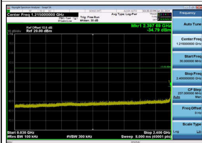
,Plot 3,30MHz~2400MHz-802.11g,2462MHz
