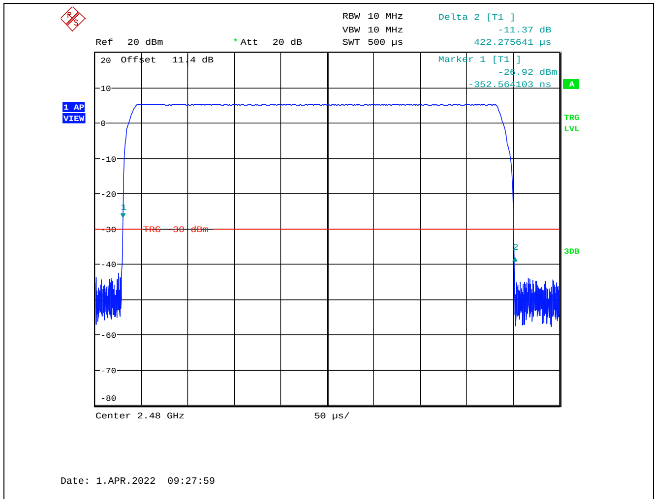
Plot 5.7.4.1.3. Duty Cycle (Pulse)
