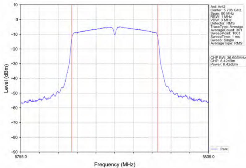
802.11n(HT40)_HCH_5795MHz_Ant2_NTNV
