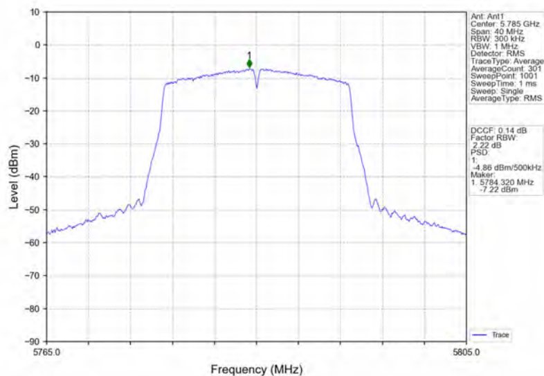
802.11n(HT20)_MCH_5785MHz_Ant1_NTNV
