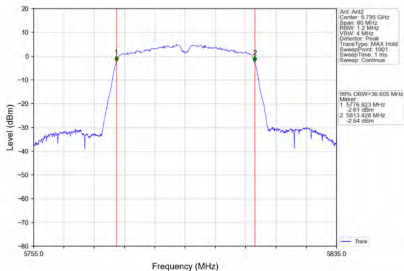
802.11n(HT40)_HCH_5795MHz_Ant2_NTNV
