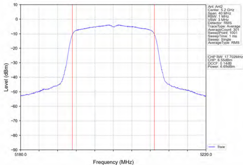
802.11n(HT20)_MCH_5200MHz_Ant2_NTNV
