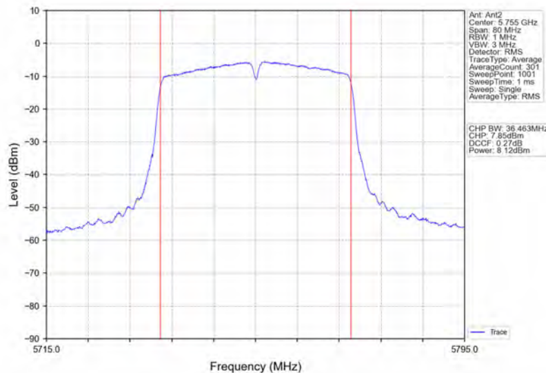
802.11ac(VHT40)_LCH_5755MHz_Ant2_NTNV
