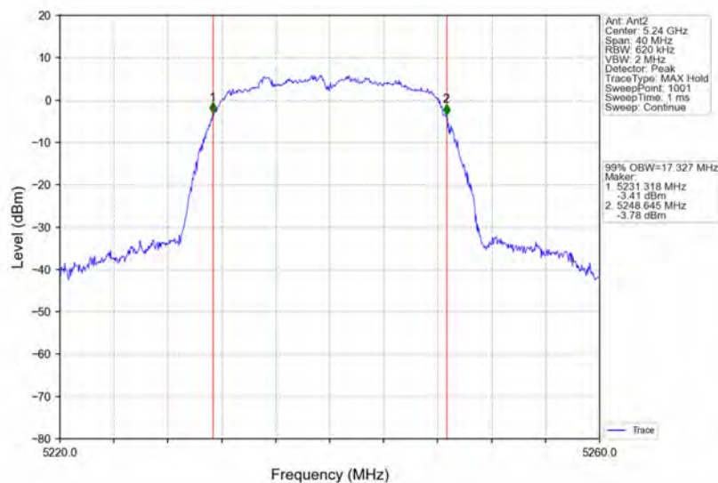
802.11a_HCH_5240MHz_Ant2_NTNV
