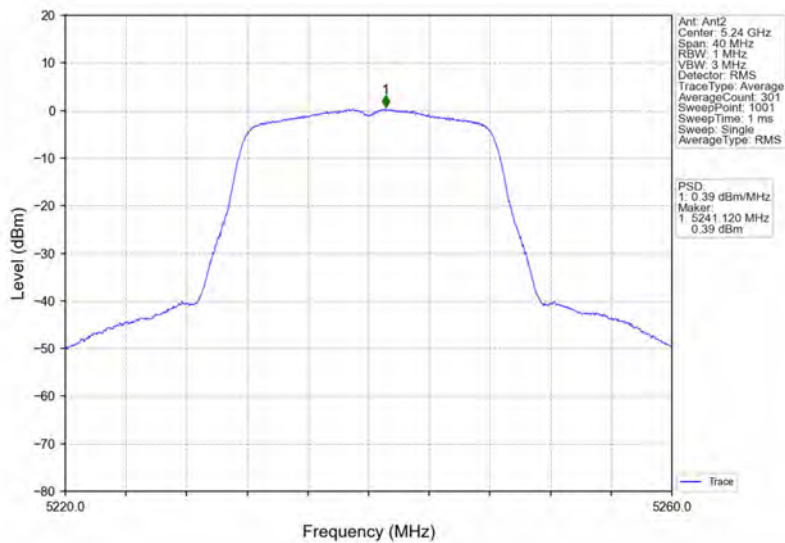
802.11a_HCH_5240MHz_Ant2_NTNV
