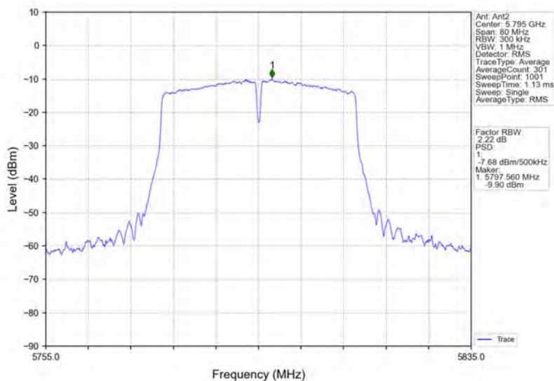
802.11n(HT40)_HCH_5795MHz_Ant2_NTNV
