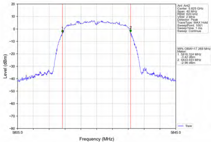
802.11a_HCH_5825MHz_Ant2_NTNV
