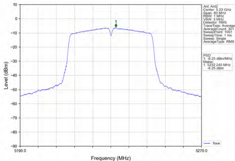
802.11n(HT40)_HCH_5230MHz_Ant2_NTNV
