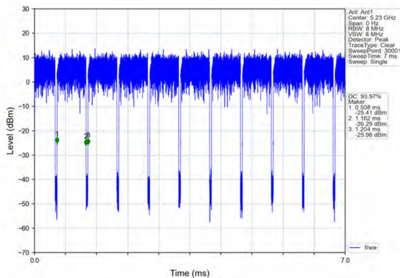
802.11ac(VHT40)_HCH_5230MHz_Ant1_NTNV
