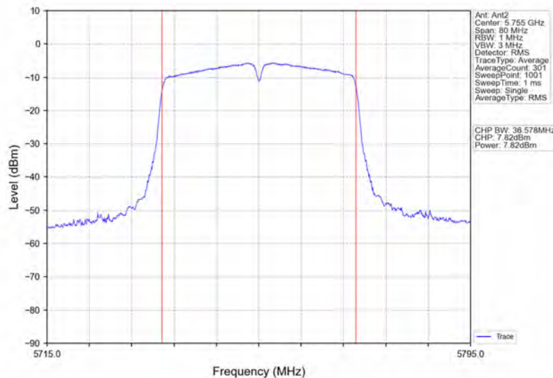
802.11n(HT40) LCH_5755MHz_Ant2_NTNV
