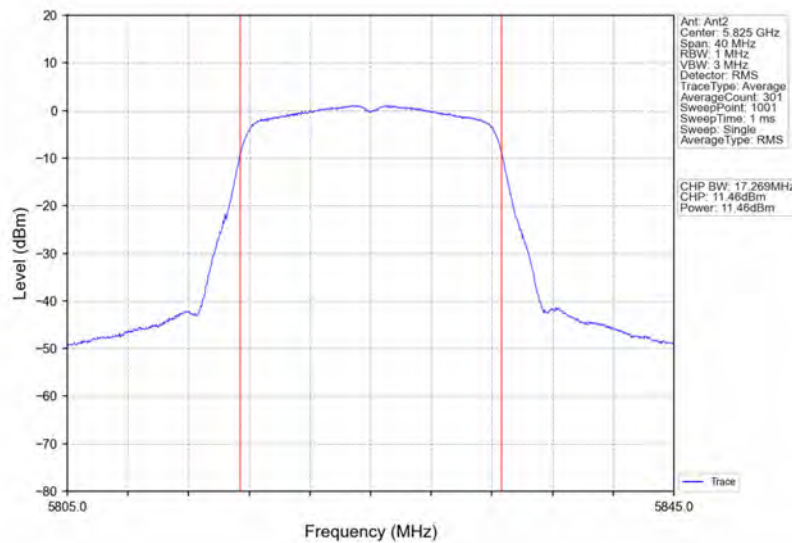
802.11a_HCH_5825MHz_Ant2_NTNV
