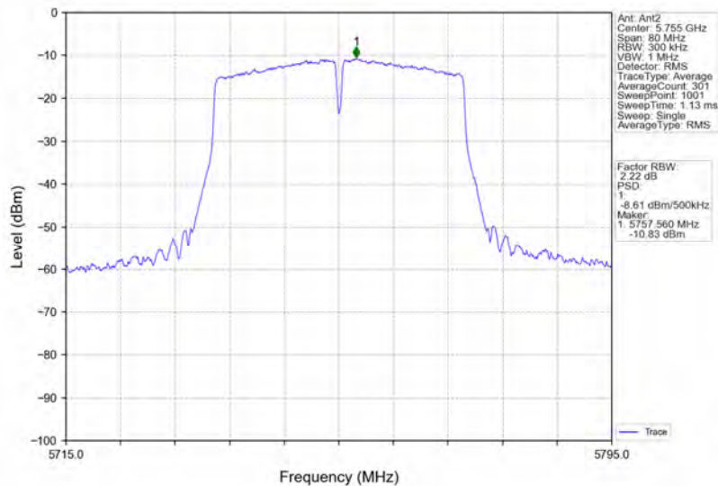
802.11n(HT40)_LCH_5755MHz_MIMO_NTNV
