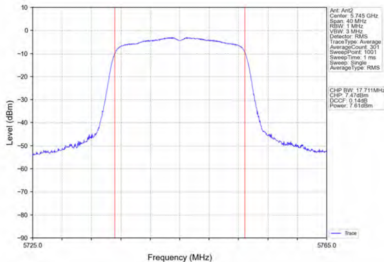
802.11n(HT20) LCH_5745MHz_Ant2_NTNV
