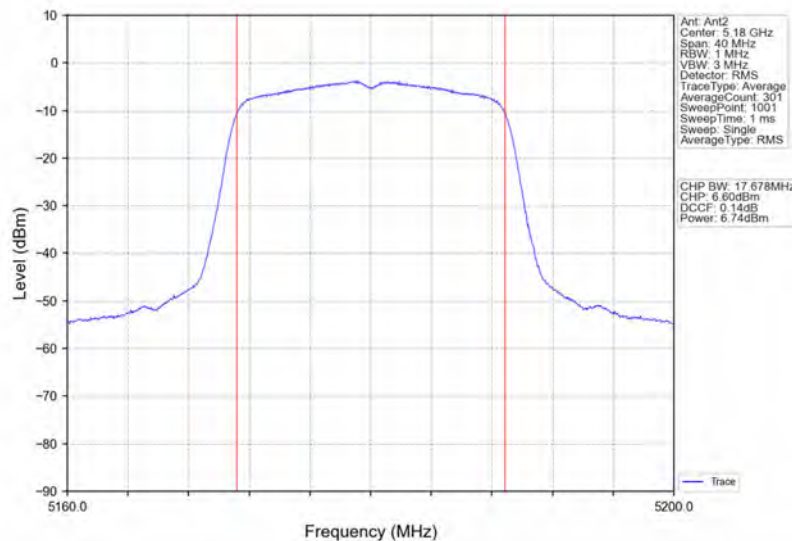
802.11n(HT20) LCH_5180MHz_Ant2_NTNV
