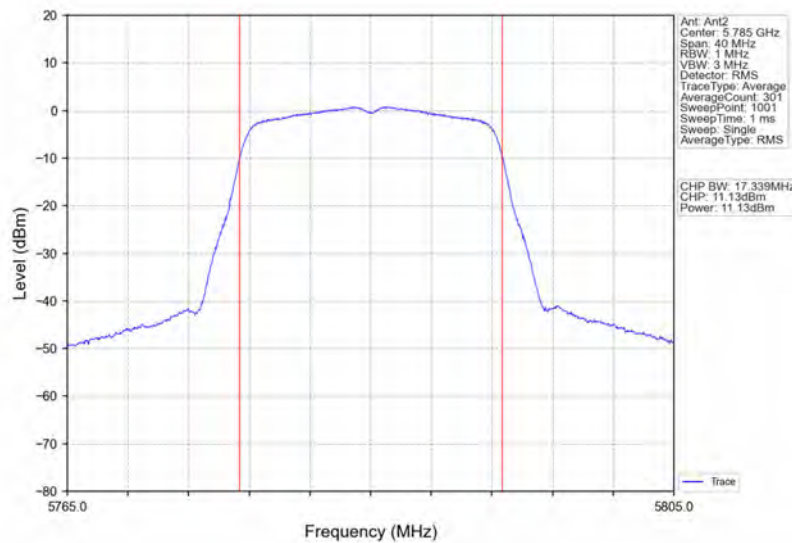
802.11a_MCH_5785MHz_Ant2_NTNV
