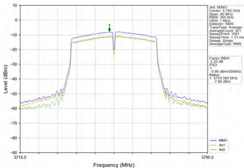
802.11n(HT40)_LCH_5755MHz_MIMO_NTNV
