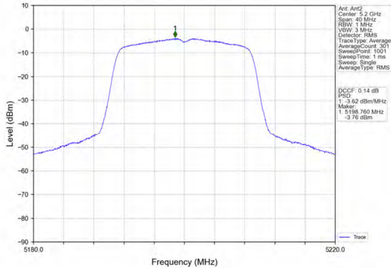
802.11n(HT20)_MCH_5200MHz_MIMO_NTNV
