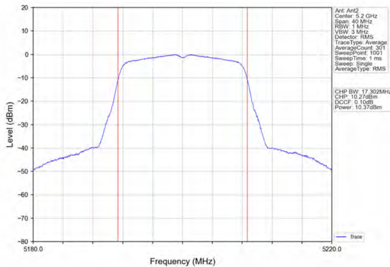
802.11a_MCH_5200MHz_Ant2_NTNV
