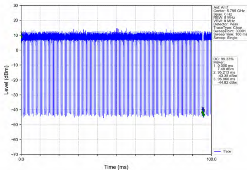
802.11n(HT40)_HCH_5795MHz_Ant1_NTNV
