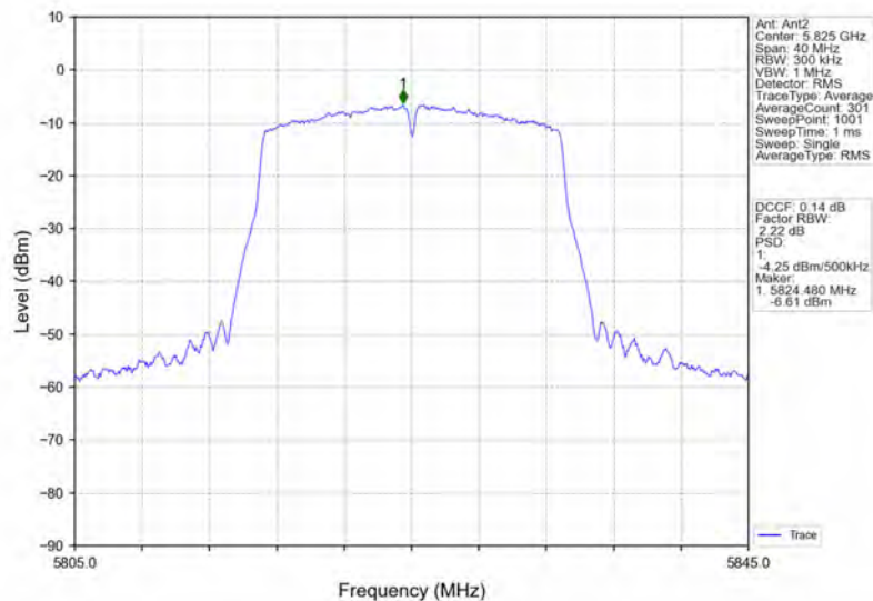
802.11n(HT20)_HCH_5825MHz_Ant2_NTNV
