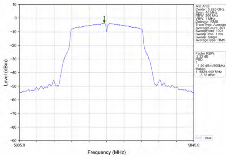
802.11a_HCH_5825MHz_Ant2_NTNV
