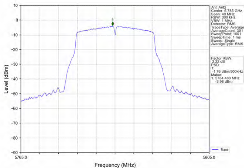
802.11a_MCH_5785MHz_Ant2_NTNV
