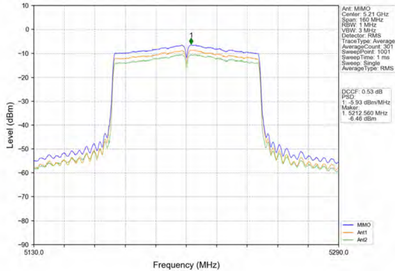
802.11ac(VHT80)_MCH_5210MHz_MIMO_NTNV
