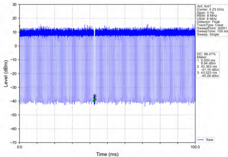
802.11n(HT40)_HCH_5230MHz_Ant1_NTNV
