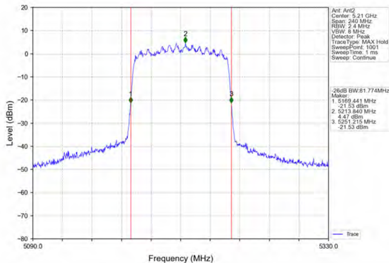
802.11ac(VHT80)_MCH_5210MHz_Ant2_NTNV
