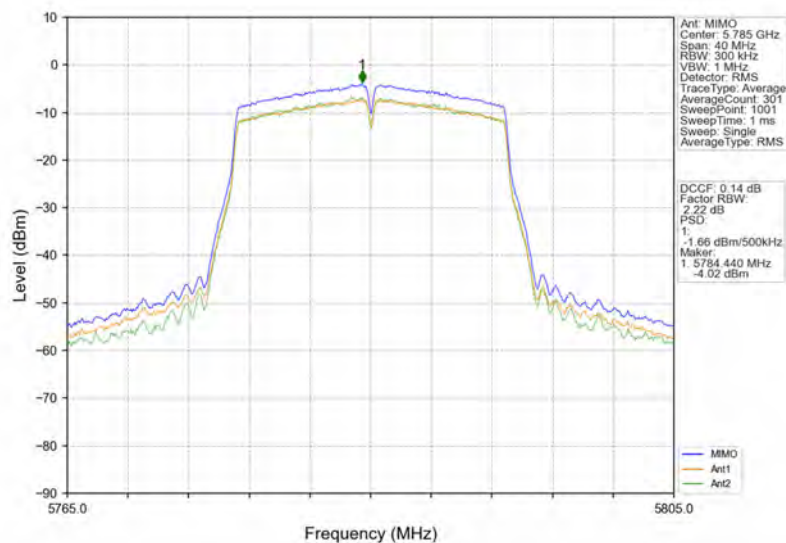
802.11n(HT20)_MCH_5785MHz_MIMO_NTNV
