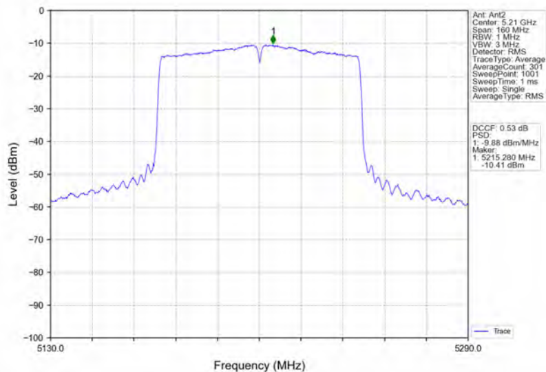
802.11ac(VHT80)_MCH_5210MHz_Ant2_NTNV
