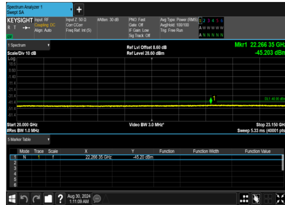
N30(5M)_DFT-s-OFDM_BPSK_Edge_1RB_Left_Low_CH
