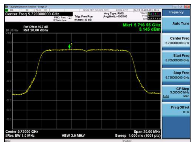
PSD-802.11n-20M-CROSS-5720M-chain4
