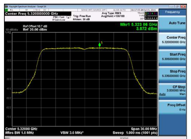
PSD-802.11n-20M-5320M-chain4
