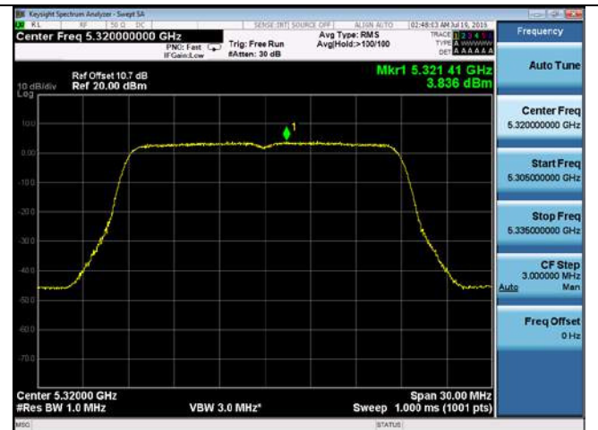
PSD-802.11n-20M-5320M-chain2
