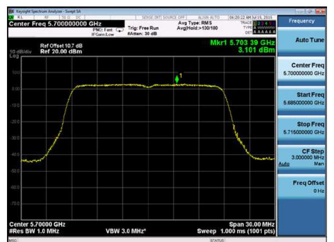
PSD-802.11n-20M-5700M-chain4
