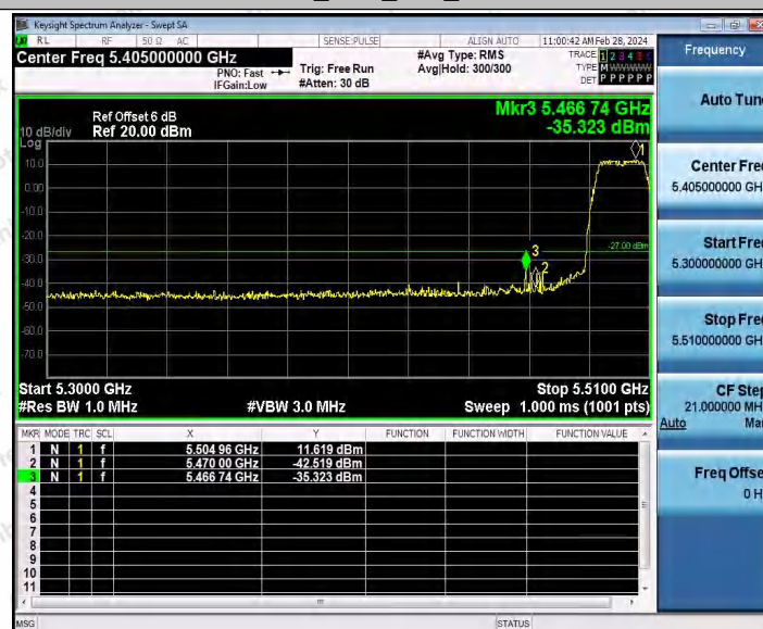
11A_Ant1_Low_5500
