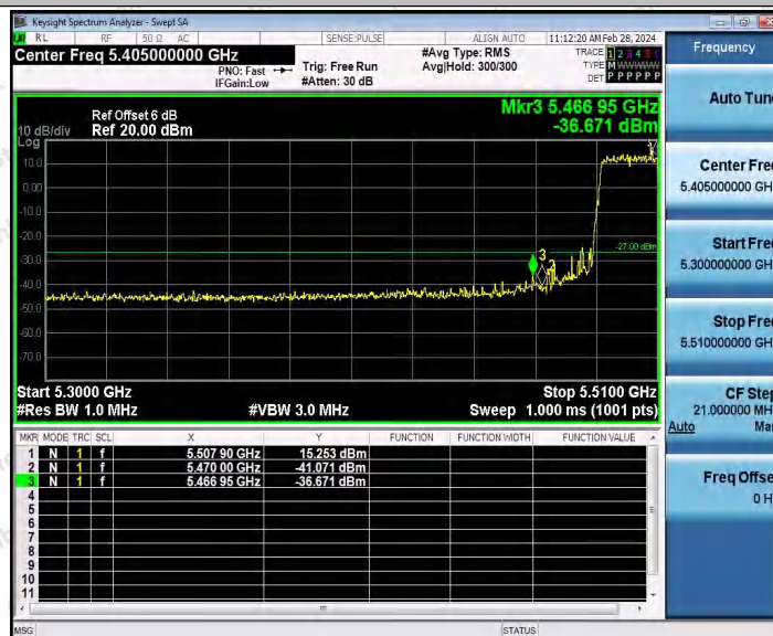
11AX20SISO_Ant1_Low_5500
