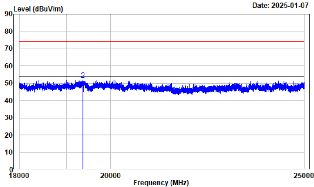
18-25GHz_Horizontal
