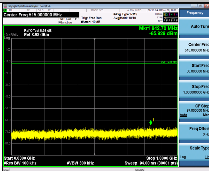
BLE_BT4.2_Ant1_2402_30~1000
