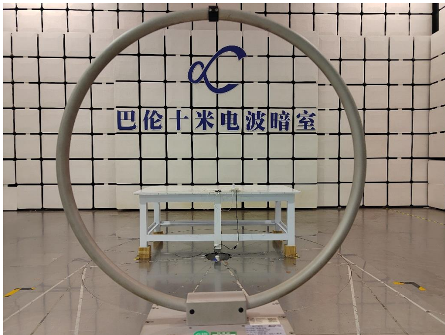
Below 30MHz-BT/WIFI
