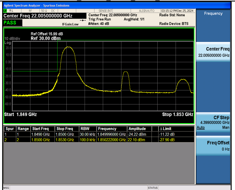
Band25 3MHz QPSK 26055 1RB#0
