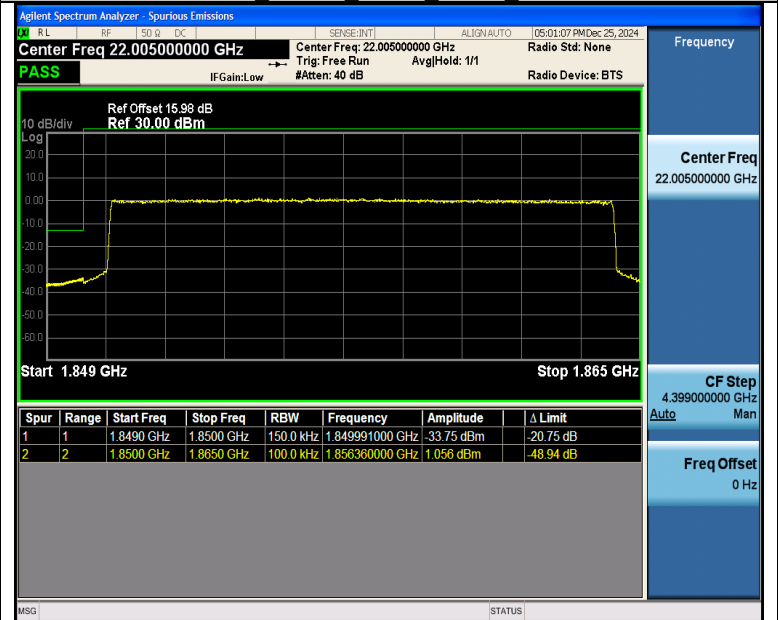
Band25 15MHz QPSK 26115 75RB#0
