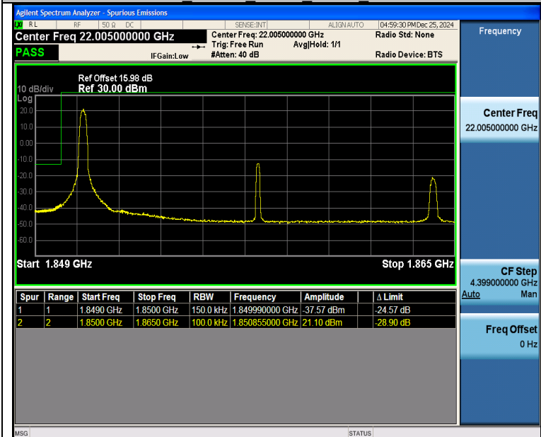
Band25 15MHz 16QAM 26115 1RB#0
