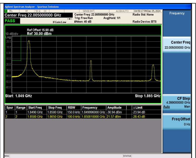
Band25 15MHz QPSK 26115 1RB#0
