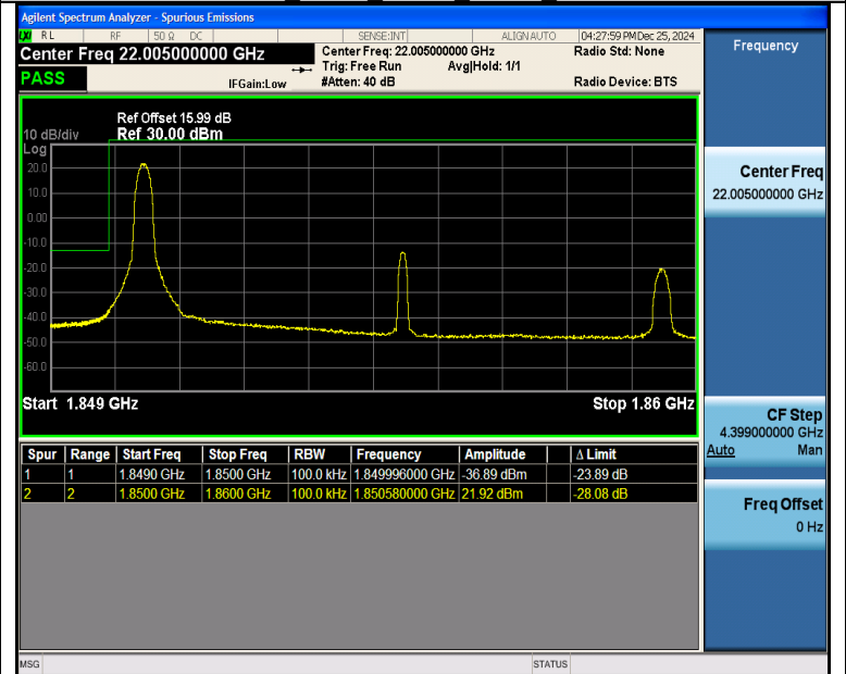
Band25 10MHz QPSK 26090 1RB#0
