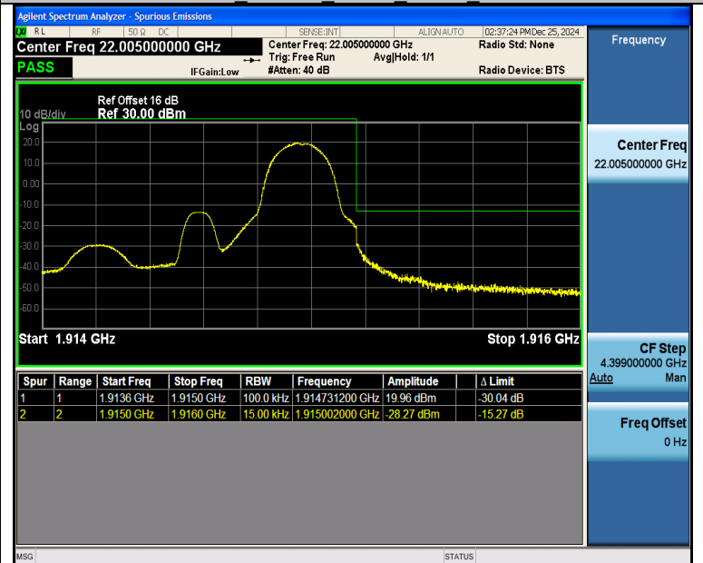
Band25 1.4MHz QPSK 26683 1RB#5
