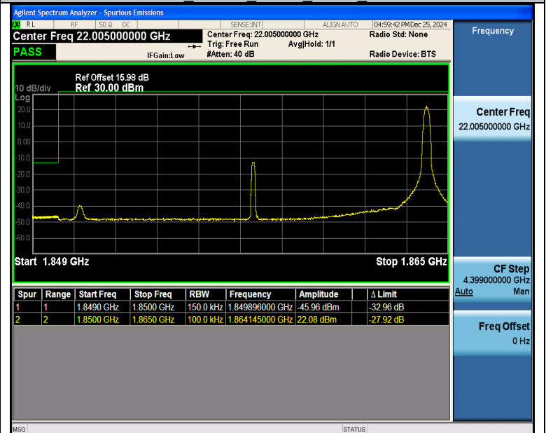
Band25 15MHz QPSK 26115 1RB#74
