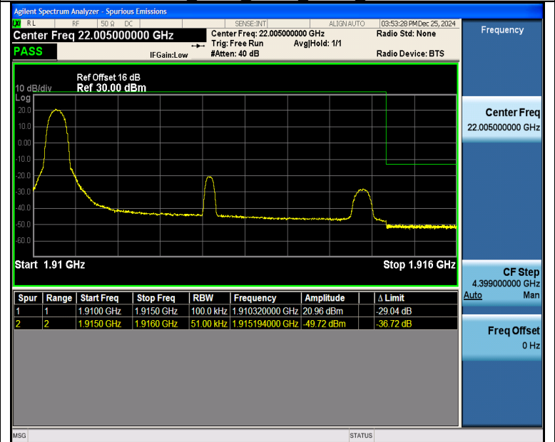
Band25 5MHz QPSK 26665 1RB#0
