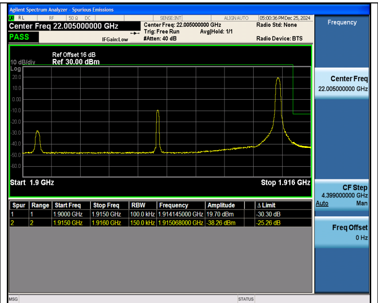
Band25 15MHz QPSK 26615 1RB#74
