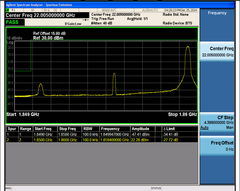
Band25 10MHz QPSK 26090 1RB#49
