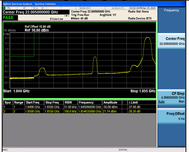
Band25 5MHz QPSK 26065 1RB#24
