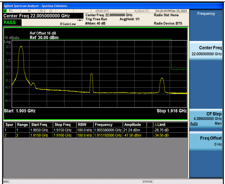
Band25 10MHz QPSK 26640 1RB#0
