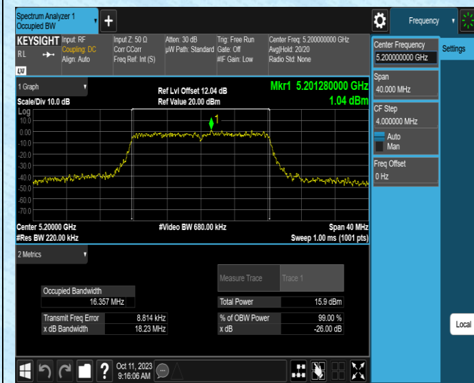
11A-Ant1-5200
