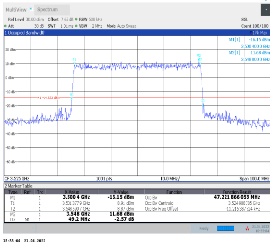
1-N78-3450-3550--30-50-H-8-CP-64QAM-Outer_Full -133@0-Ant0-47.222-49.200-≤50-PASS
