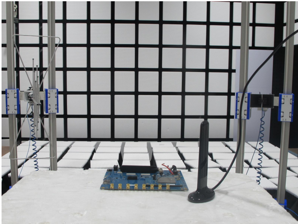
RSE_30MHz-18GHz
