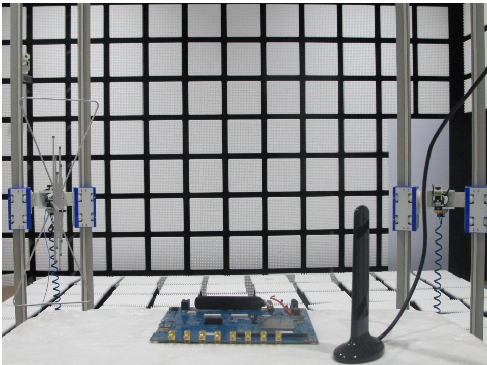
RSE_18GHz-20GHz
