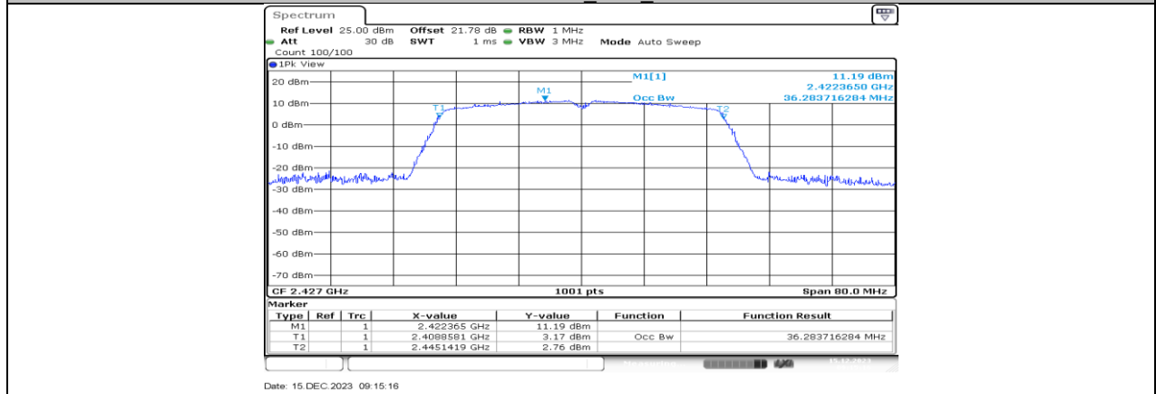
11N40MIMO_Ant1_2427
