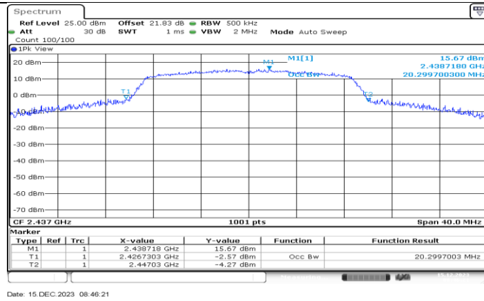
11N20MIMO_Ant1_2437
