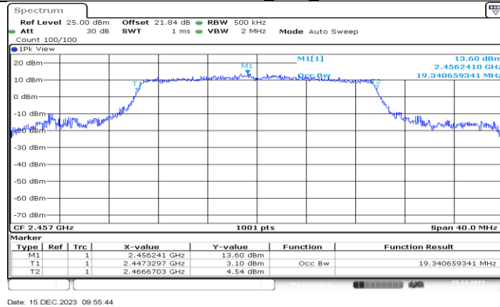
11AX20MIMO_Ant1_2457
