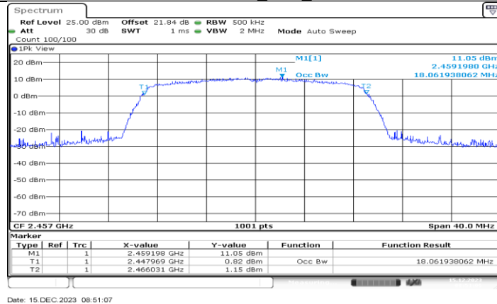
11N20MIMO_Ant1_2457
