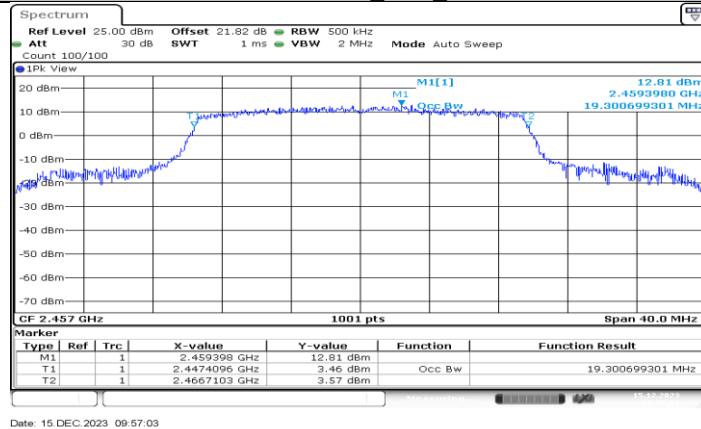
11AX20MIMO_Ant2_2457
