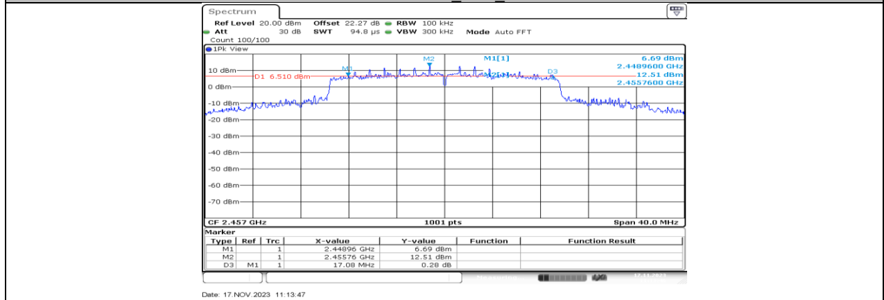
11AX20MIMO_Ant2_2457
