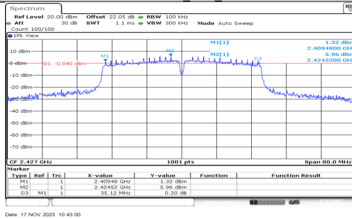
11N40MIMO_Ant1_2427
