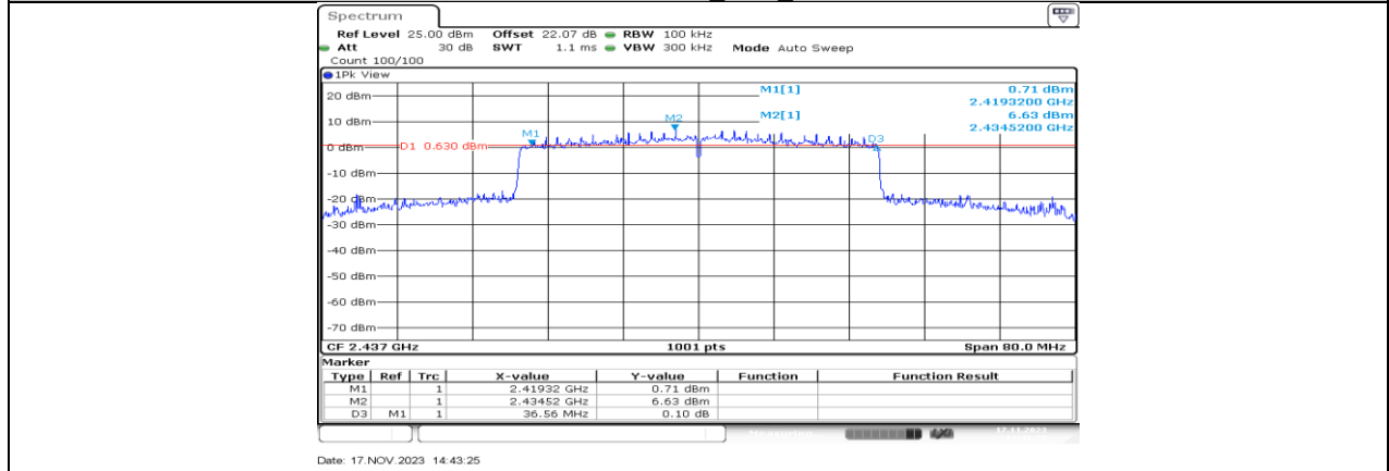
11AX40MIMO_Ant1_2437
