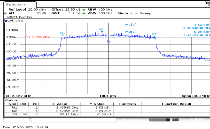
11N40MIMO_Ant2_2427
