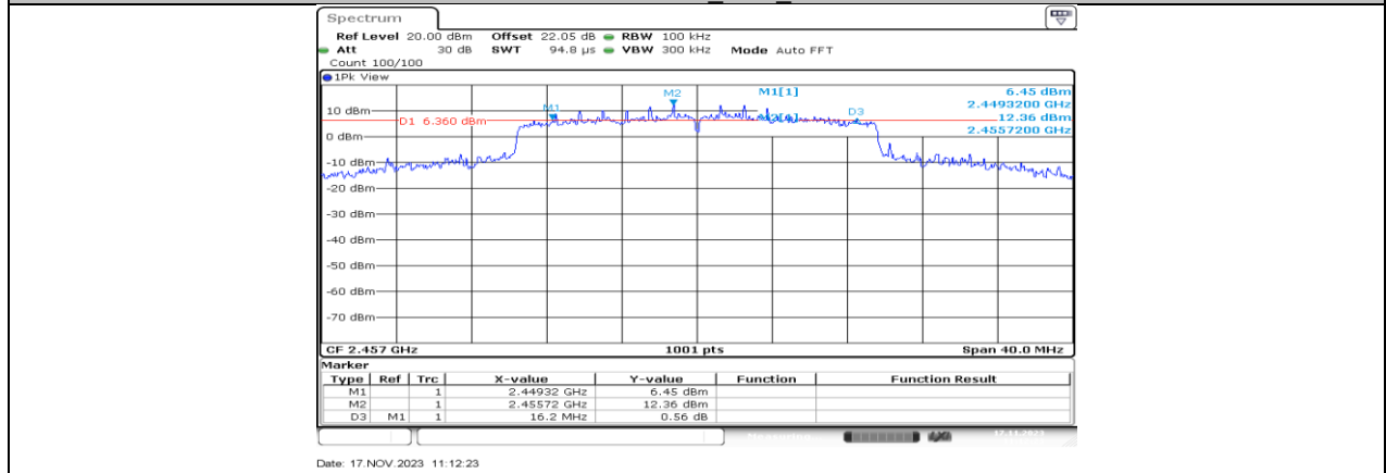
11AX20MIMO_Ant1_2457
