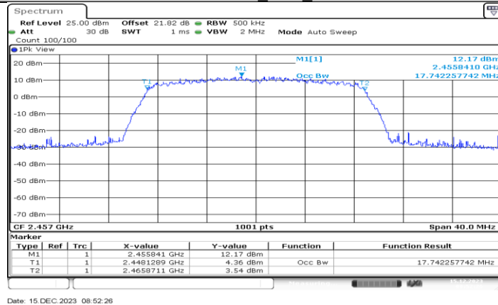
11N20MIMO_Ant1_2457
