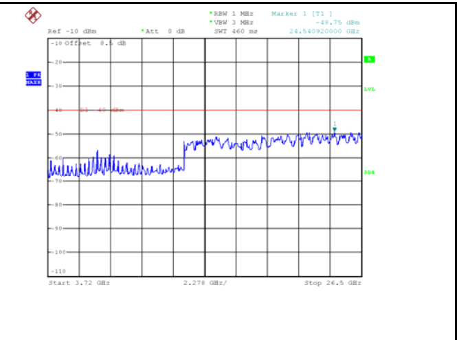
5MHz - High CH 3.72GHz~26.5GHz
